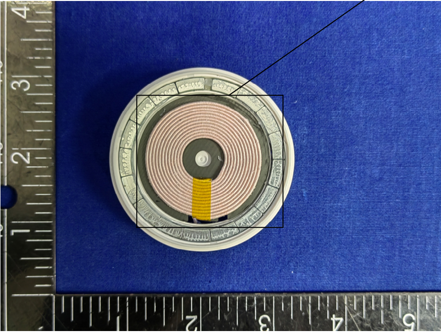
WPT1 Ant
