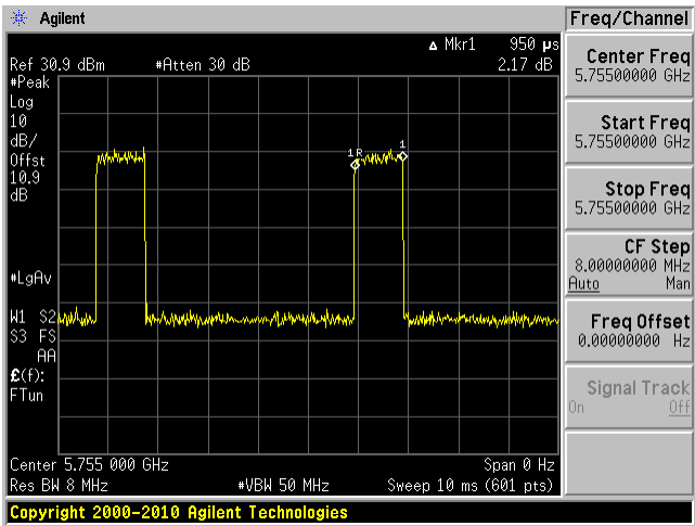
802.11ac40 mode Pulse Width
