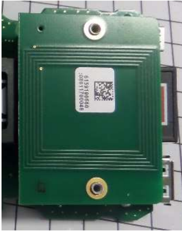
RFID antenna
