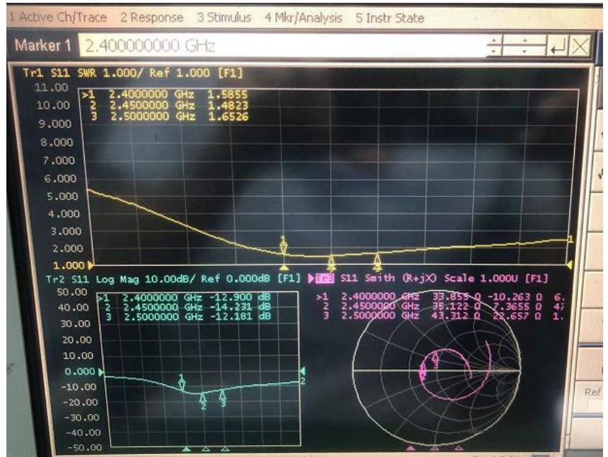
天线性能测试图:
