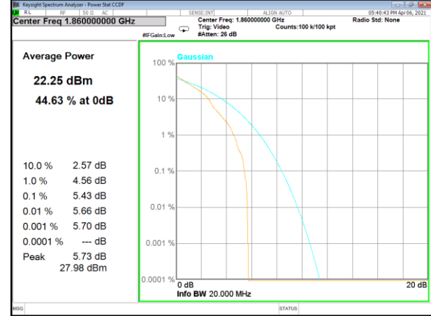
Band 25_1_Q16_Low
