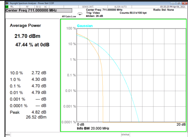
Band 12_1_Q16_High
