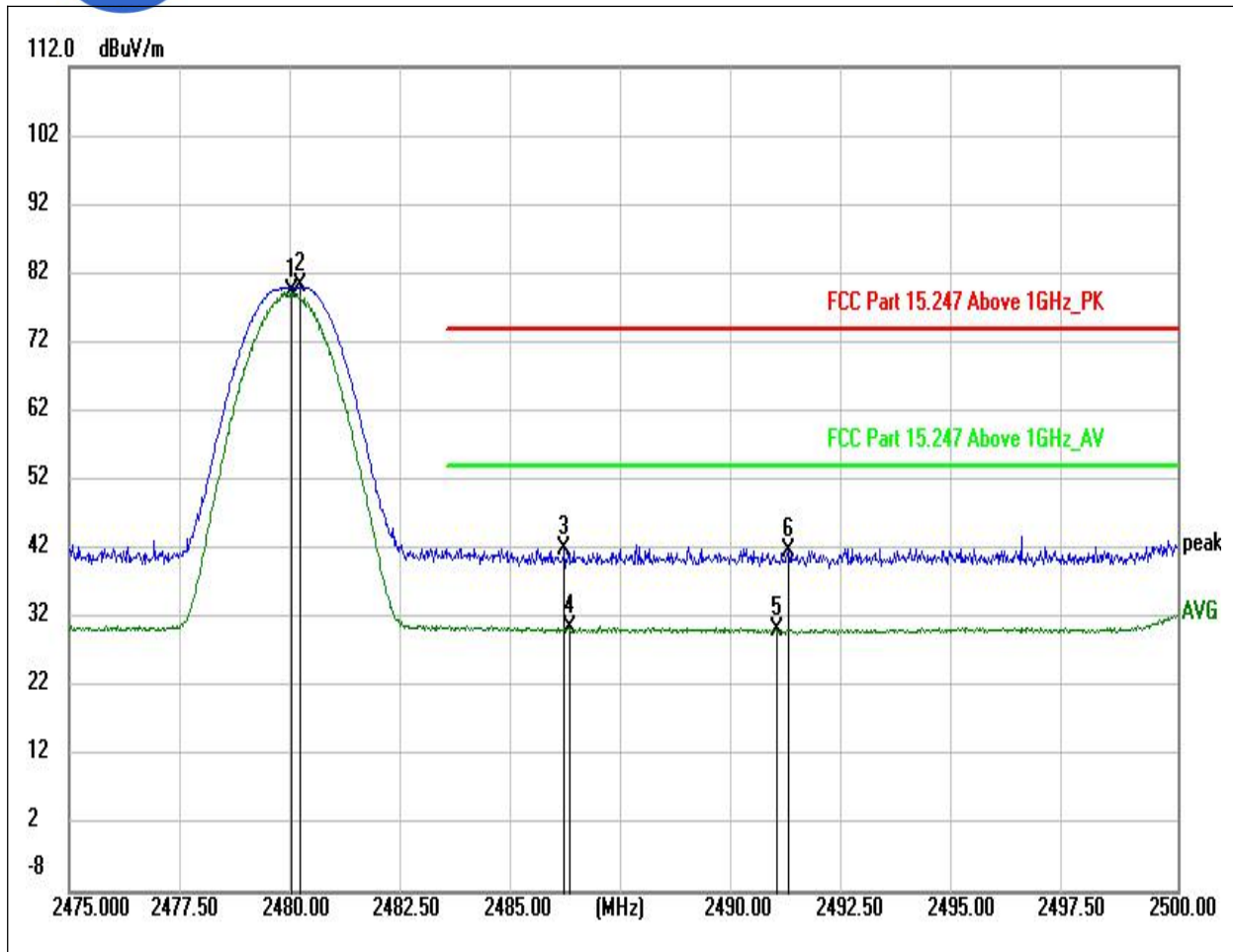
(LE 1M PHY_2480MHz, Antenna Horizontal)
