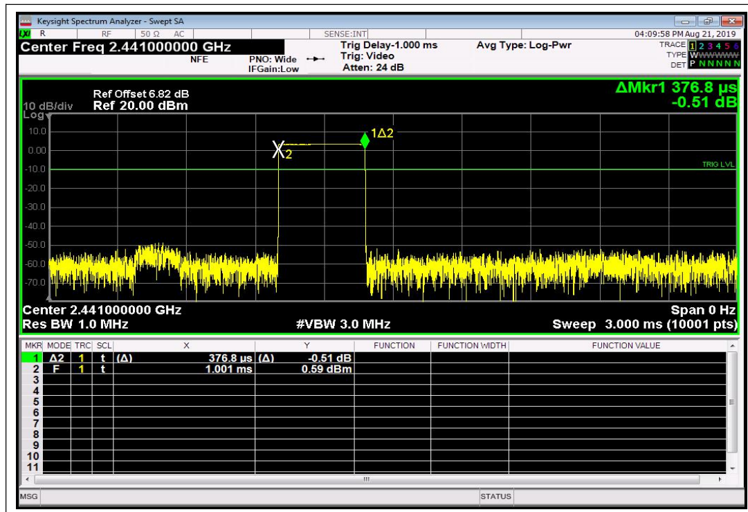
(DH1_2441M, GFSK)
