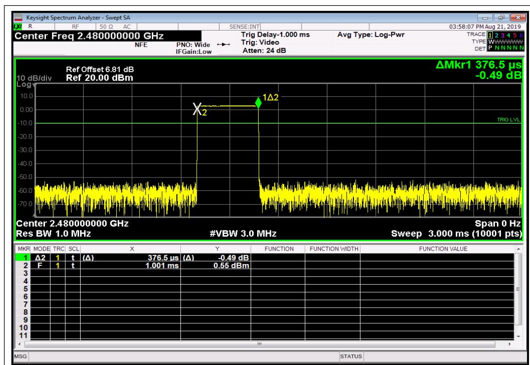
(DH1_2480M, GFSK)
