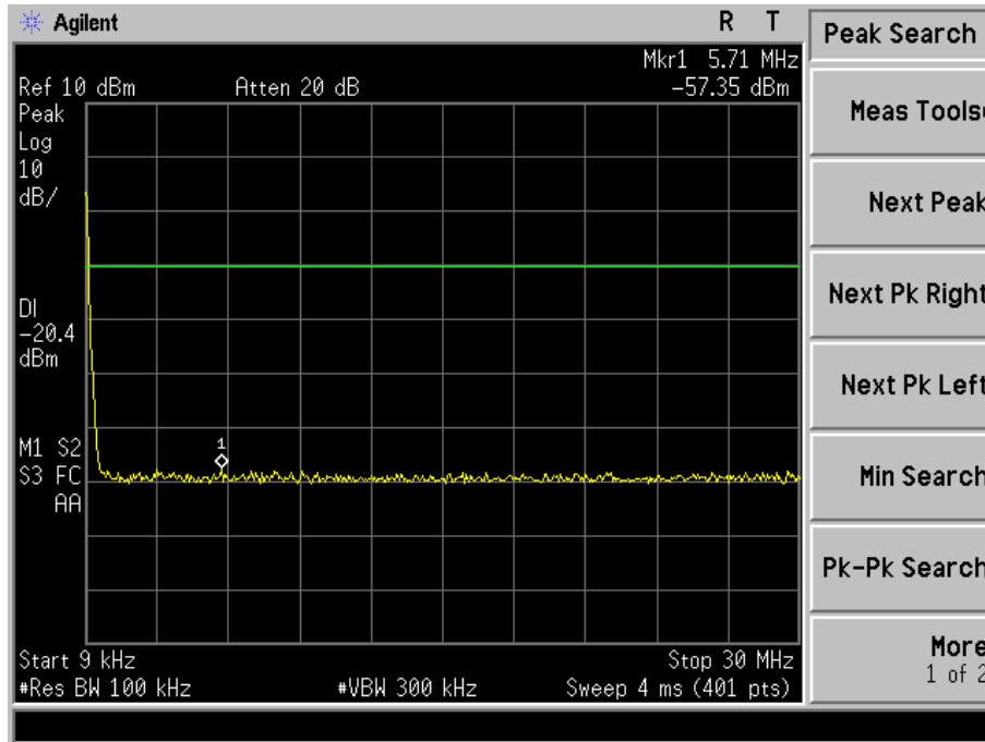
9KHz - 30MHz 802.11b Low Channel
