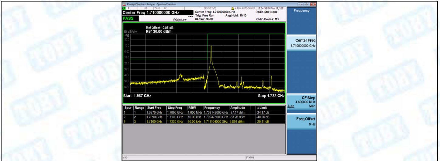
Band4-20MHz-QPSK-20050-1RB#99
