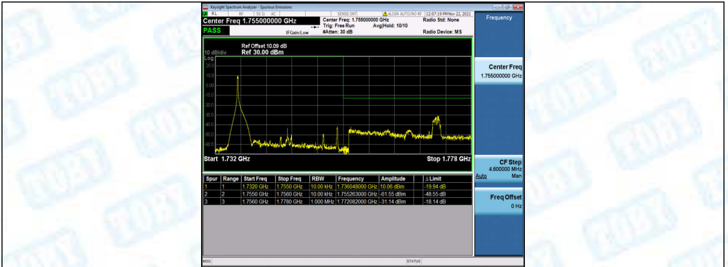
Band4-20MHz-QPSK-20300-1RB#99
