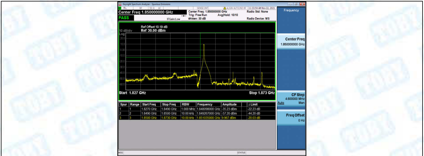
Band2-20MHz-QPSK-18700-1RB#99
