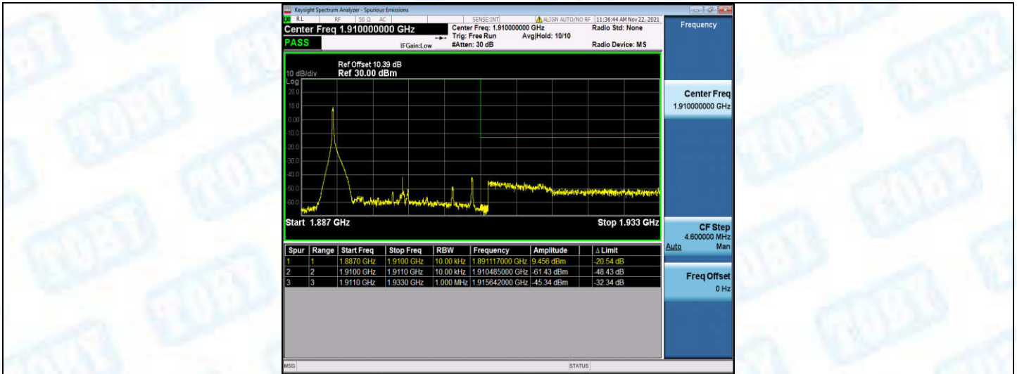
Band2-20MHz-16QAM-19100-1RB#99
