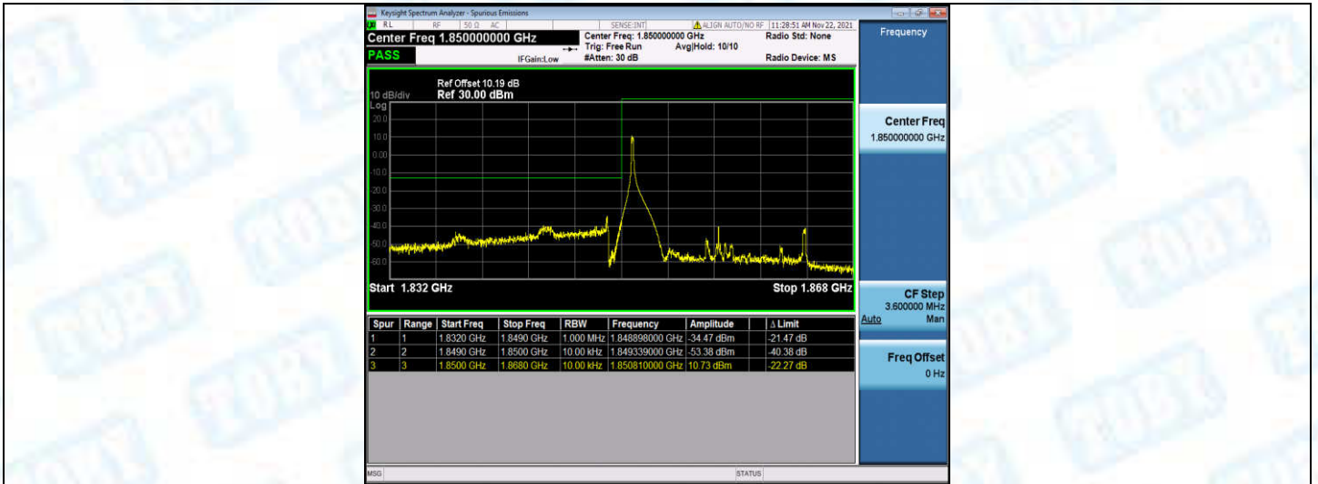
Band2-15MHz-16QAM-18675-1RB#74
