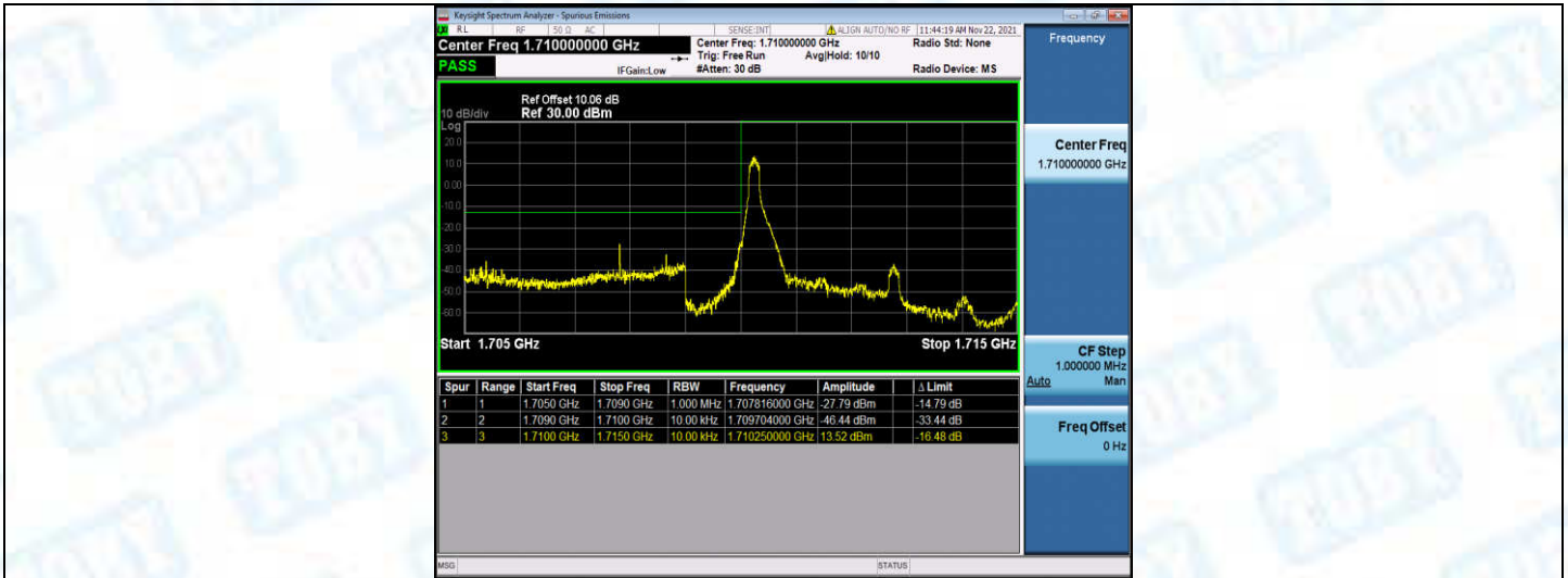
Band4-3MHz-QPSK-19965-1RB#14
