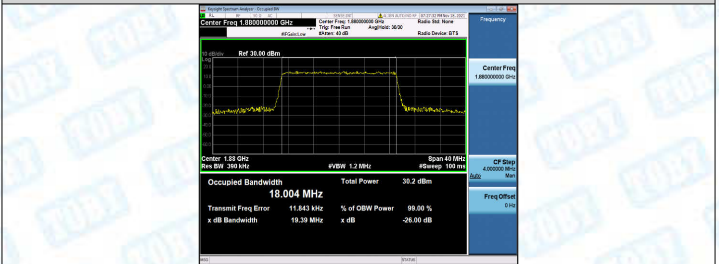
Band2-20MHz-16QAM-19100-100RB#0
