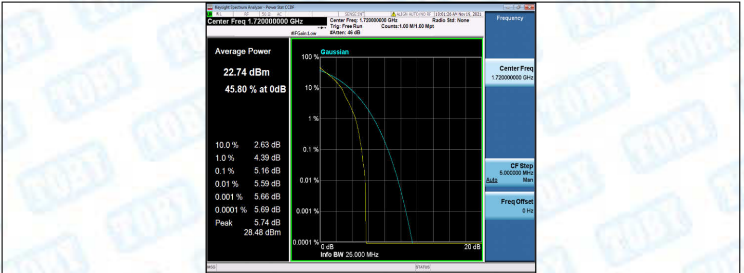
Band4-20MHz-QPSK-20050-100RB#0
