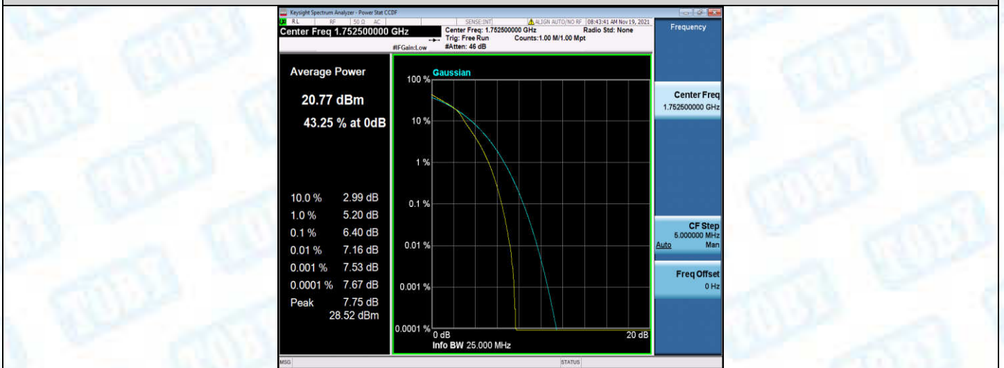
Band4-10MHz-QPSK-20000-1RB#0
