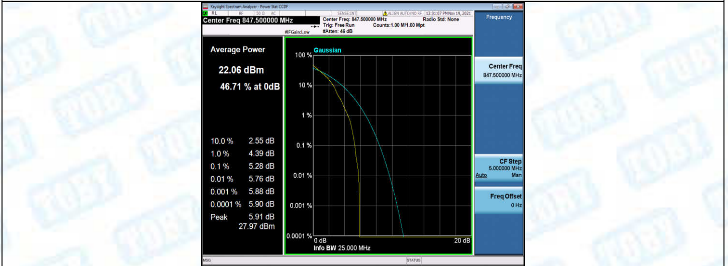
Band5-3MHz-QPSK-20635-15RB#0
