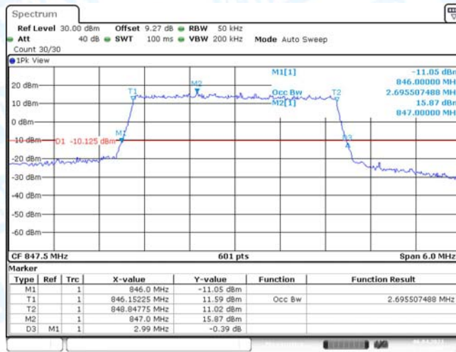
Band5-3MHz-QPSK-20635-15RB#0
