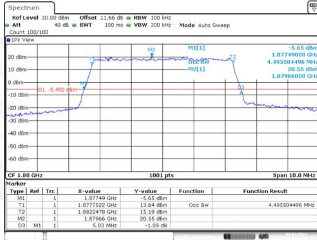
Band2-5MHz-QPSK-18900-25RB#0
