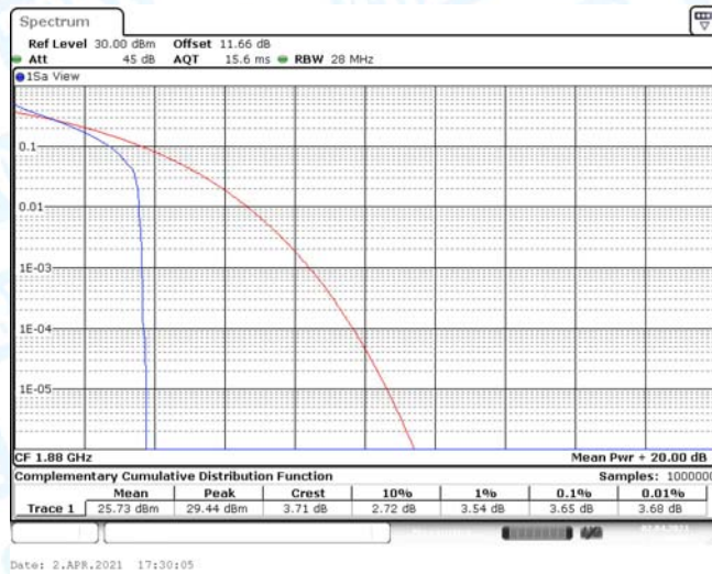
Band2-10MHz-QPSK-18900-50RB#0
