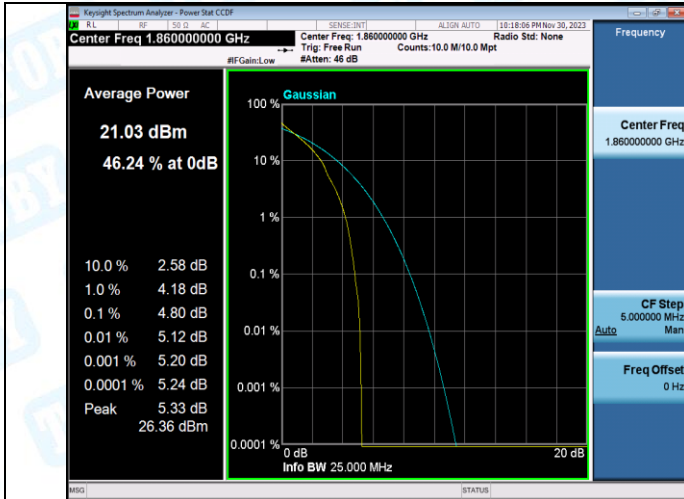
Band2-20MHz-QPSK-18700-100RB#0-PASS
