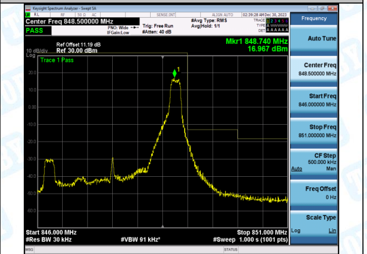
Band5_3MHz_16QAM_20635_15RB#0
