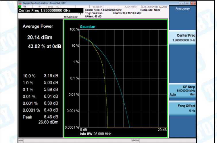
Band2-20MHz-16QAM-18700-100RB#0-PASS
