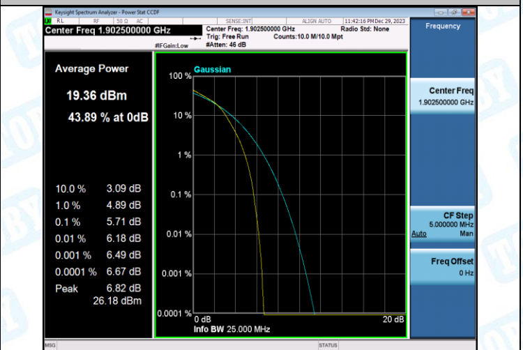
Band2-20MHz-16QAM-18700-1RB#0-PASS
