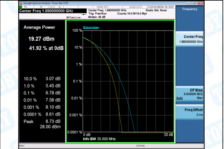
Band2-20MHz-16QAM-19100-1RB#0-PASS
