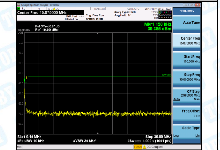
Band4-1513-5-1000~20000MHz-PASS
