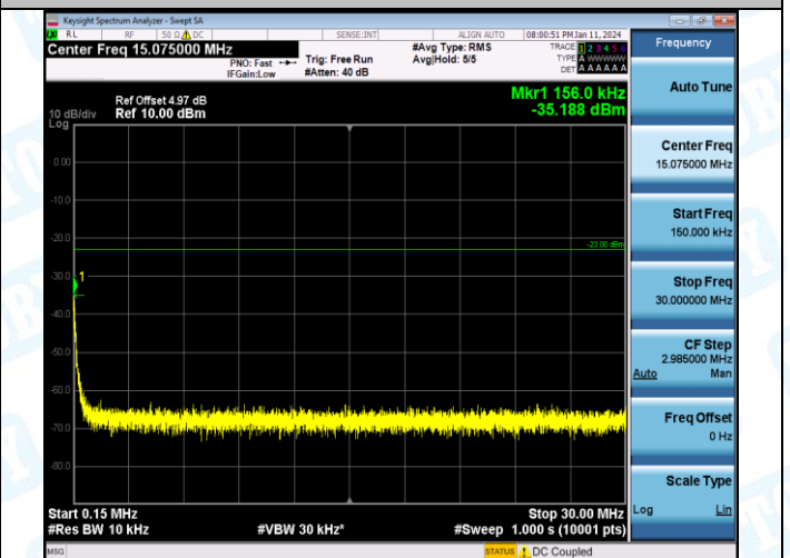
GSM1900-512-0-0.15~30MHz-PASS
