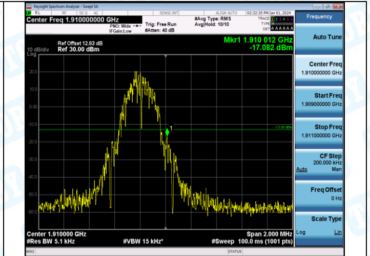
EGPRS1900-810-2-PASS
