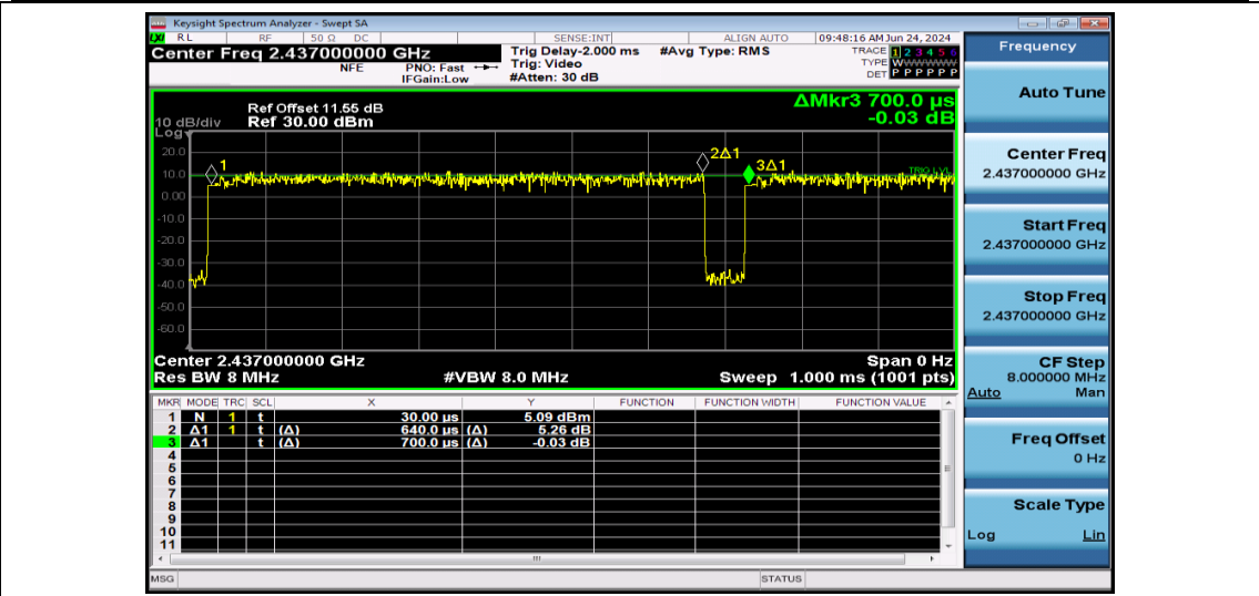
NTNV-11N40MIMO-Ant2-2437
