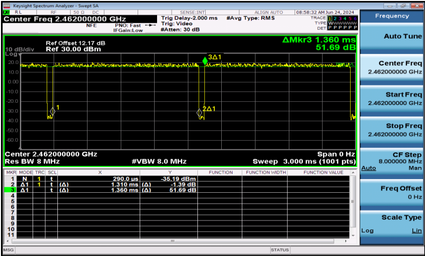
NTNV-11N20MIMO-Ant1-2462
