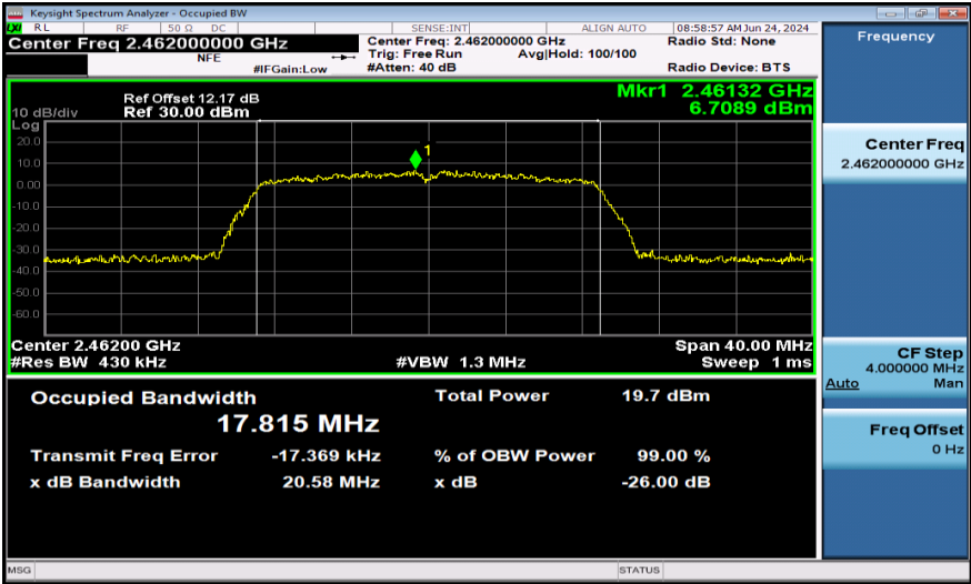
11N20MIMO-Ant1-2462
