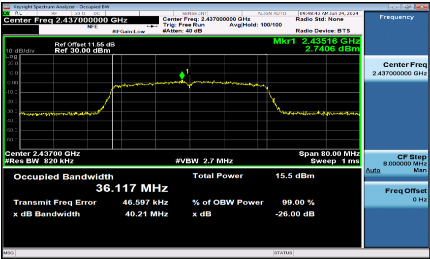
11N40MIMO-Ant2-2437
