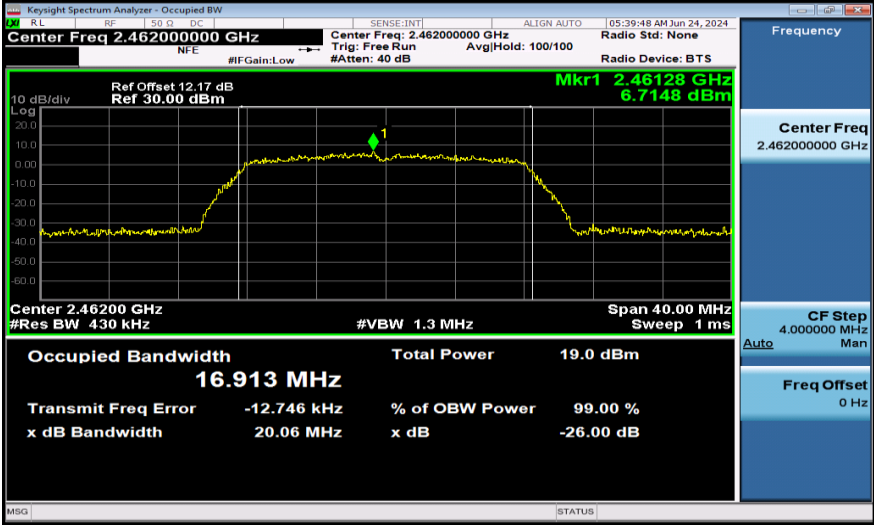
11G-Ant1-2462
