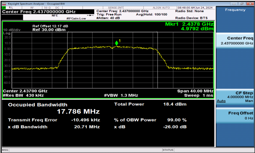
11N20MIMO-Ant1-2437
