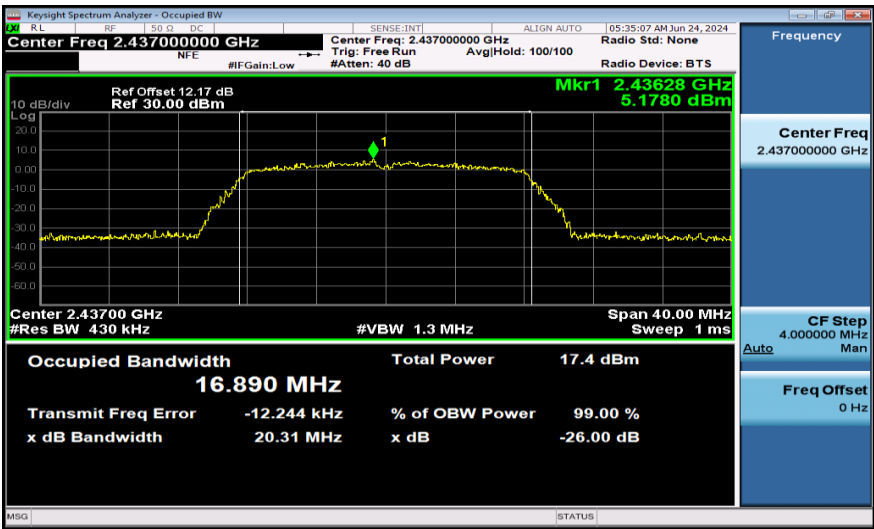
11G-Ant1-2437
