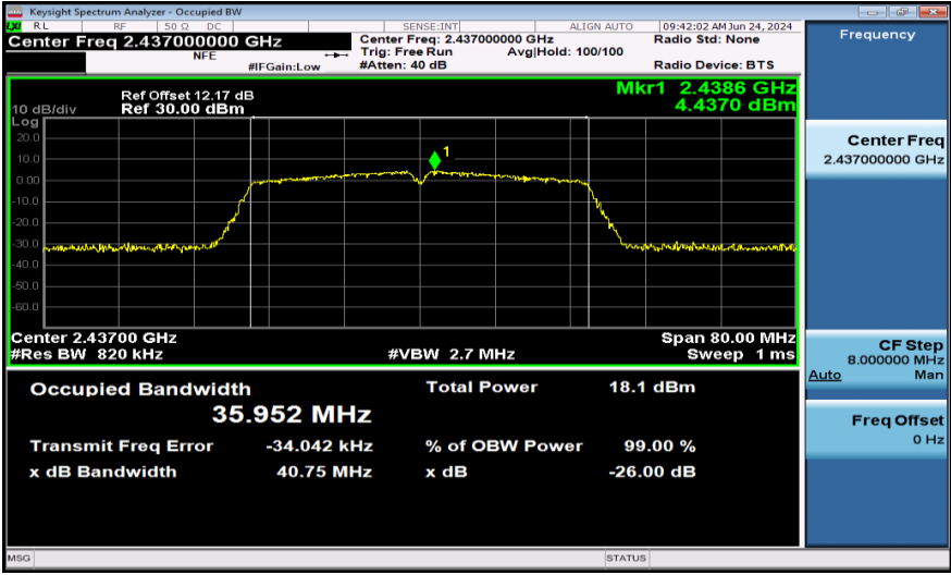
11N40MIMO-Ant1-2437
