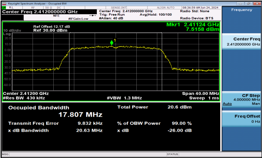
11N20MIMO-Ant1-2412
