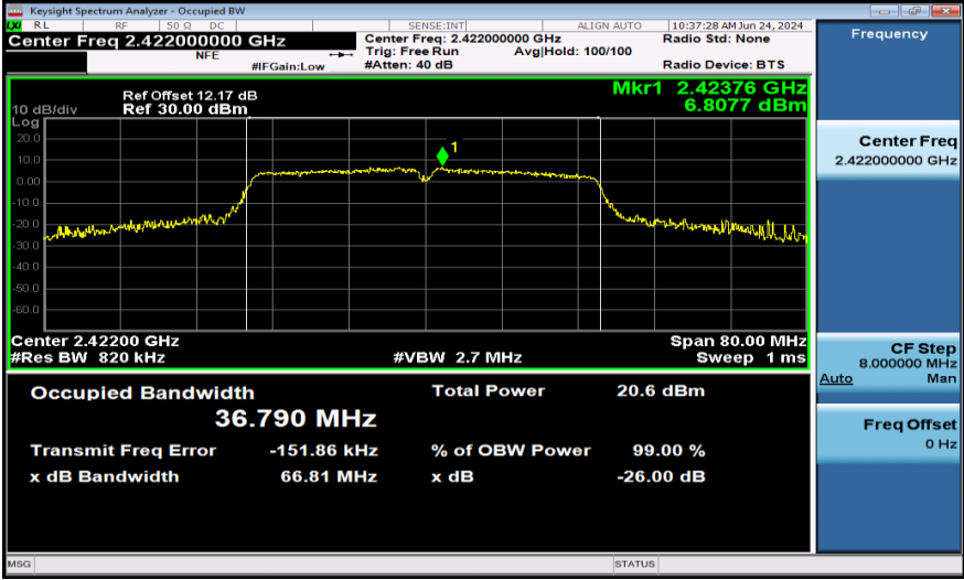
11N40MIMO-Ant1-2422
