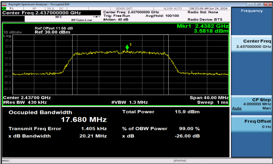
11N20MIMO-Ant2-2437
