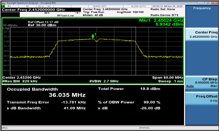
11N40MIMO-Ant1-2452
