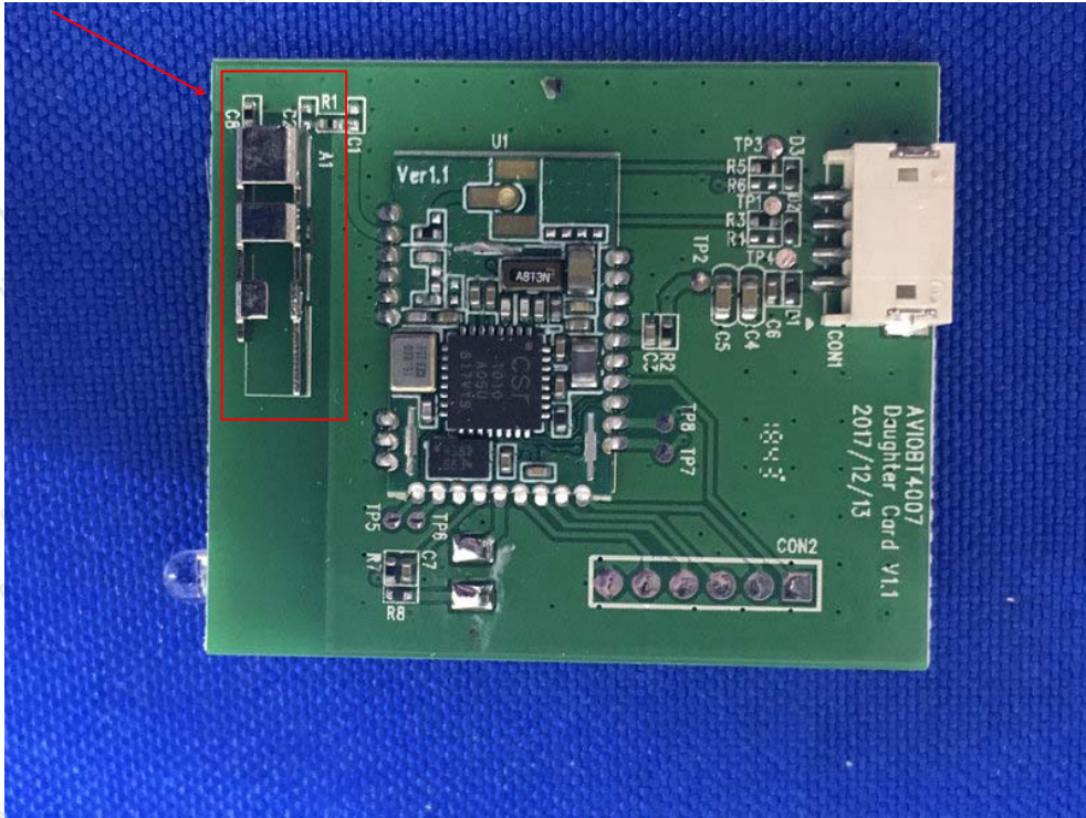
BLE module 2
