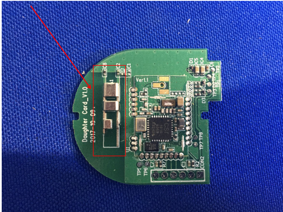
BLE module 1 antenna
