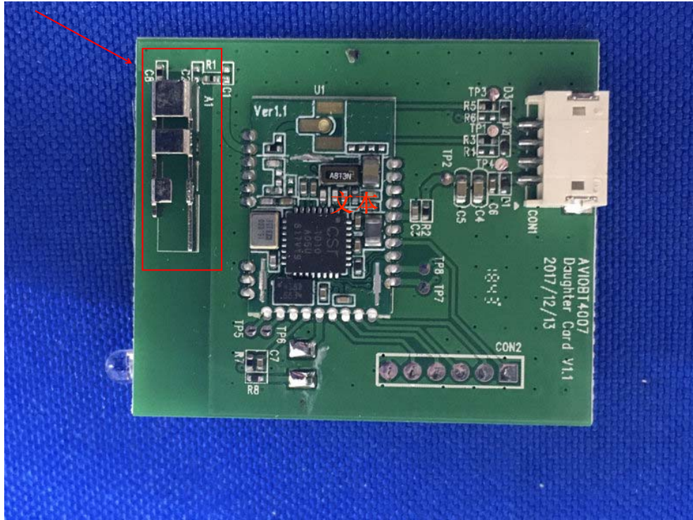
BLE module 2 antenna
