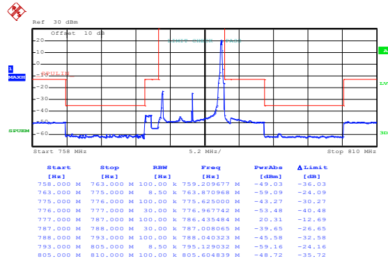
QPSK & RB Size 49
