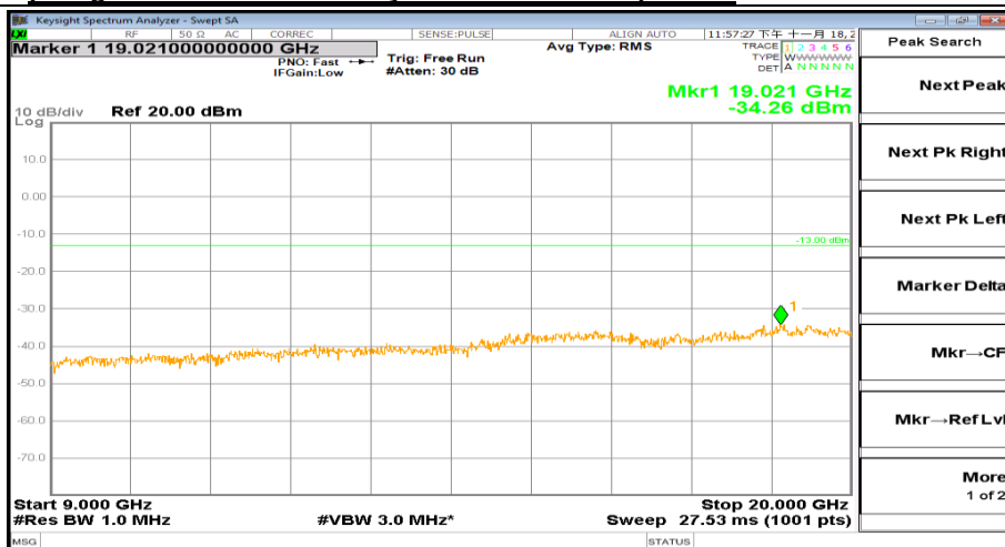
9000MHz-20000MHz_FreqMid_BW( 20MHz)_RB(1@0)_QPSK_Band25
