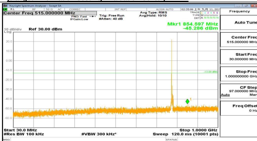
30MHz-1000MHz_FreqMid_BW( 5MHz)_RB(1@0)_QPSK_Band13
