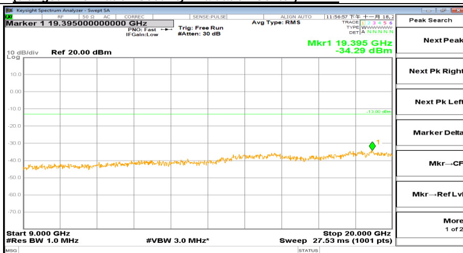
9000MHz-20000MHz_FreqLow_BW( 20MHz)_RB(1@0)_QPSK_Band25
