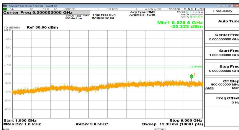
1000MHz-9000MHz_FreqMid_BW( 10MHz)_RB(1@0)_QPSK_Band13
