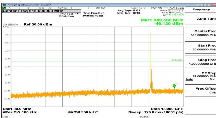
30MHz-1000MHz_FreqMid_BW( 5MHz)_RB(1@0)_QPSK_Band26
