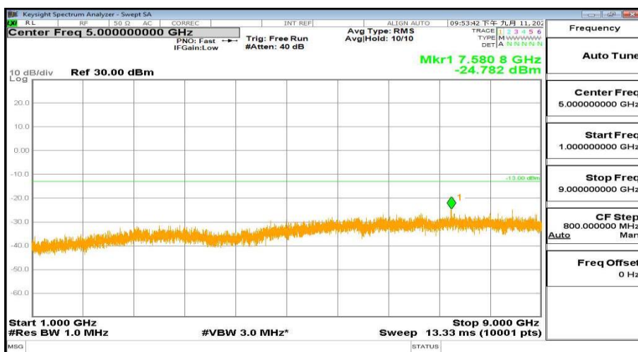
1000MHz-9000MHz_FreqMid_BW( 10MHz)_RB(1@0)_QPSK_Band26
