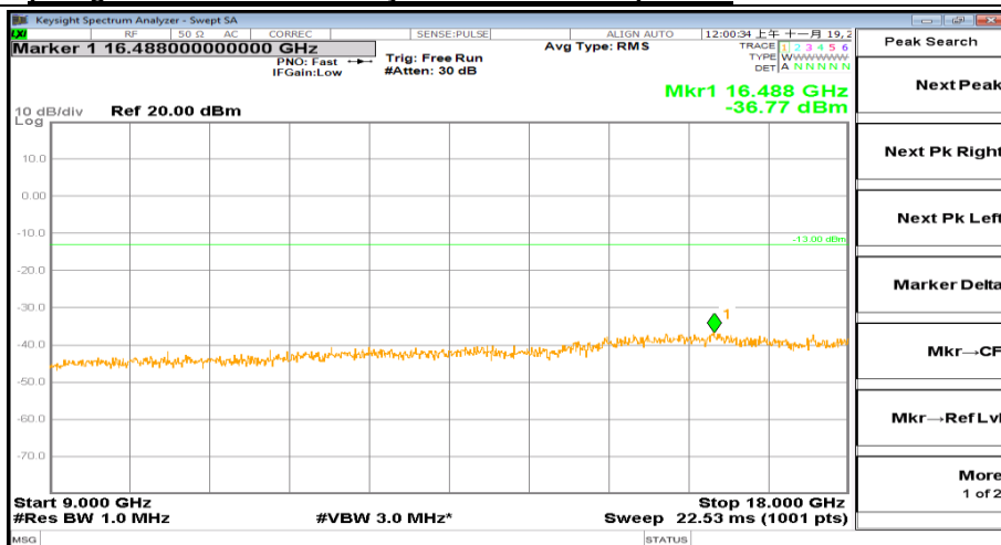
9000MHz-18000MHz_FreqMid_BW(_3MHz)_RB(1@0)_QPSK_Band4
