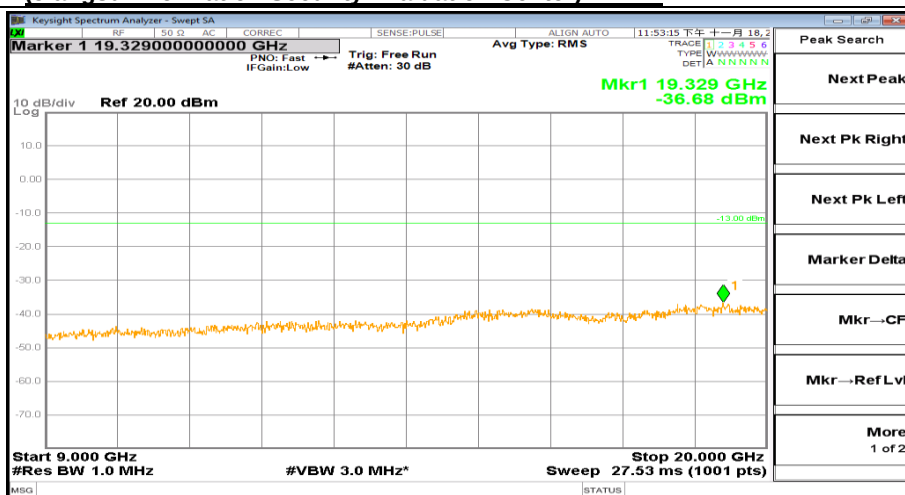
9000MHz-20000MHz_FreqLow_BW(_20MHz)_RB(1@0)_QPSK_Band2
