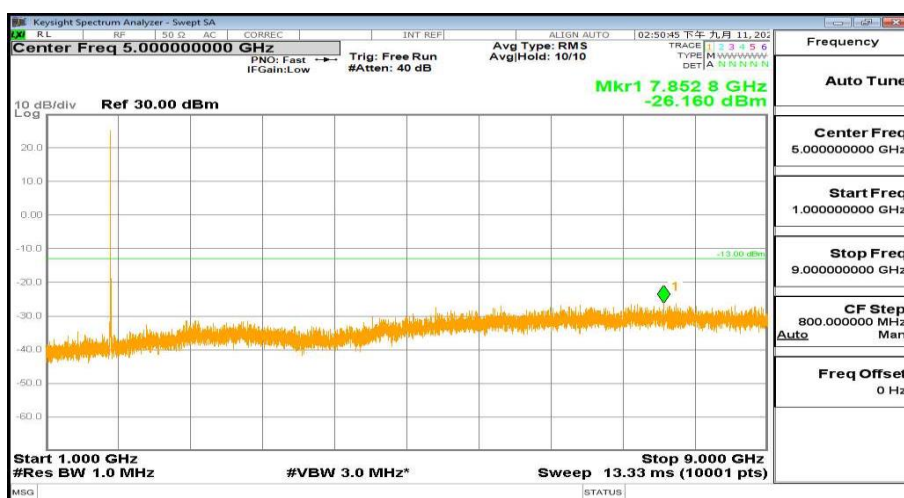
1000MHz-9000MHz_FreqLow_BW( 10MHz)_RB(1@0)_QPSK_Band4
