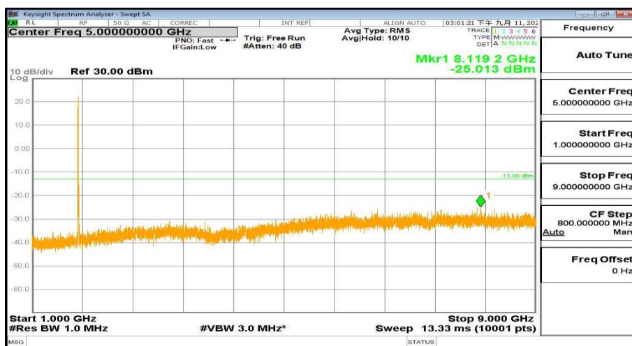
1000MHz-9000MHz_FreqMid_BW(_10MHz)_RB(1@0)_QPSK_Band4
