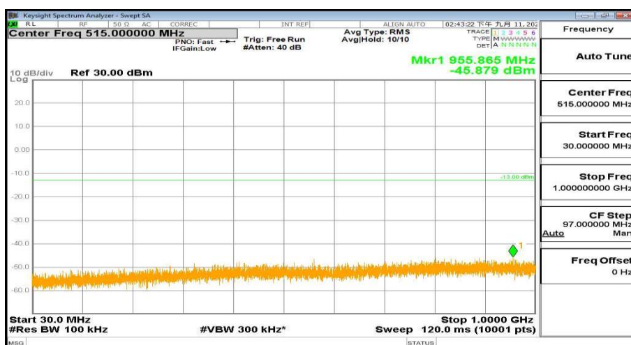
30MHz-1000MHz_FreqLow_BW( 5MHz)_RB(1@0)_QPSK_Band4
