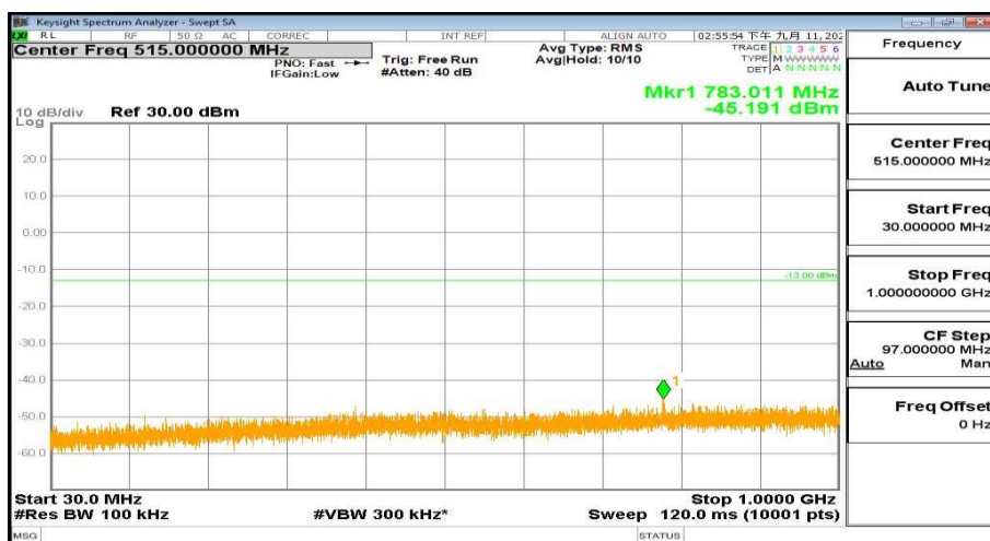
30MHz-1000MHz_FreqMid_BW(_5MHz)_RB(1@0)_QPSK_Band4
