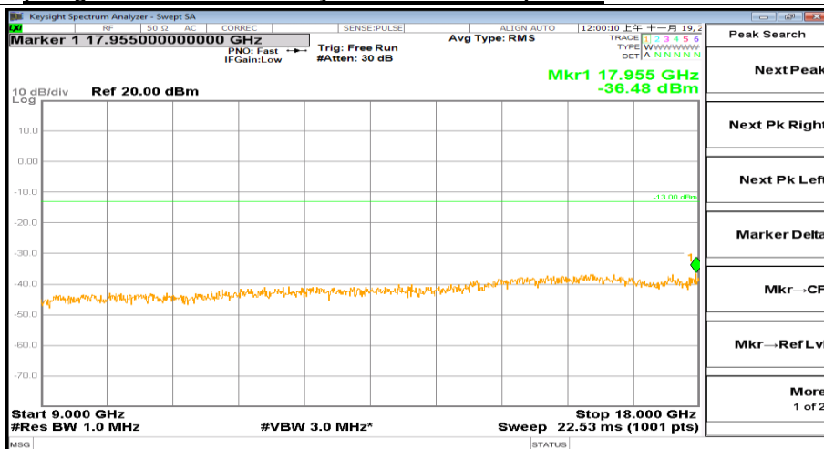
9000MHz-18000MHz_FreqLow_BW( 3MHz)_RB(1@0)_QPSK_Band4
