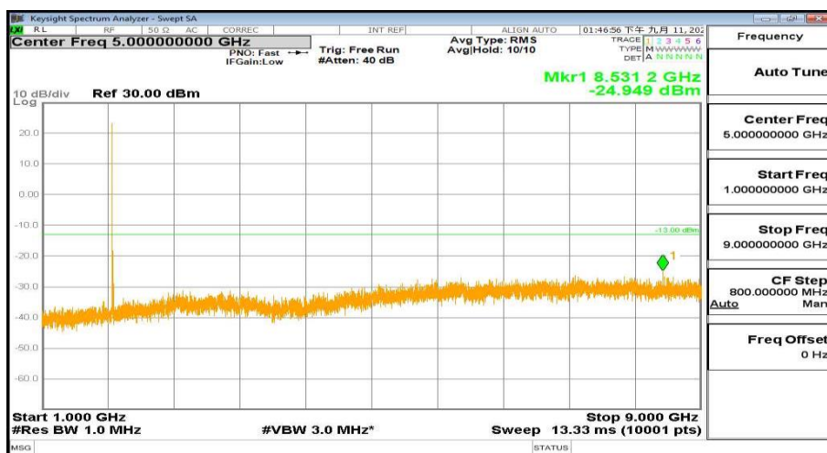
1000MHz-9000MHz_FreqLow_BW( 10MHz)_RB(1@0)_QPSK_Band2
