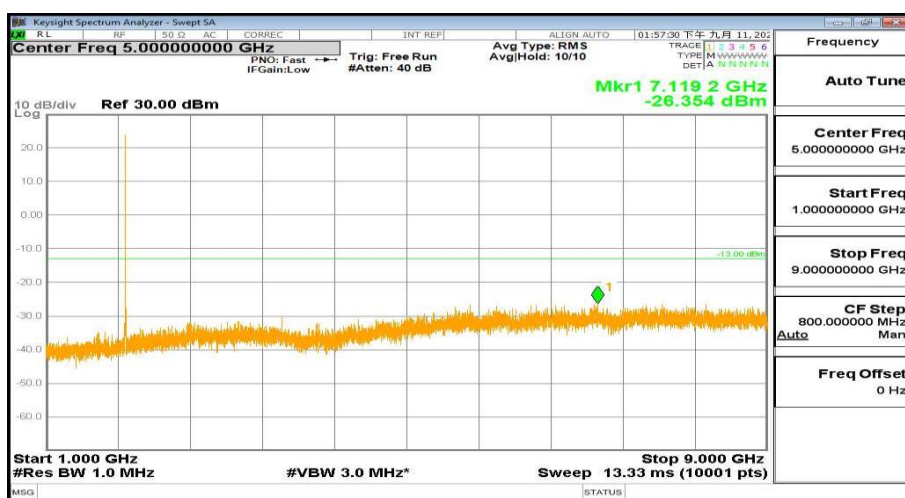
1000MHz-9000MHz_FreqMid_BW(_3MHz)_RB(1@0)_QPSK_Band2
