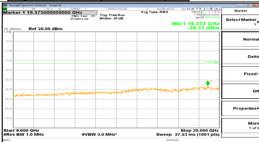
9000MHz-20000MHz_FreqLow_BW( 3MHz)_RB(1@0)_QPSK_Band2
