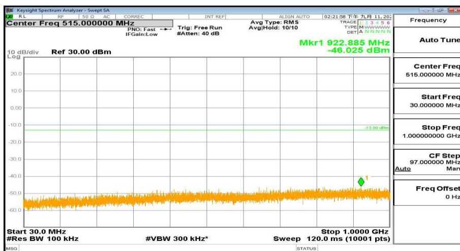
30MHz-1000MHz_FreqLow_BW( 5MHz)_RB(1@0)_QPSK_Band2
