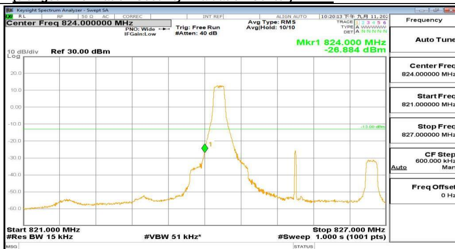
821MHz-827MHz_FreqLow_BW(_3MHz)_RB(1@0)_QPSK_Band26
