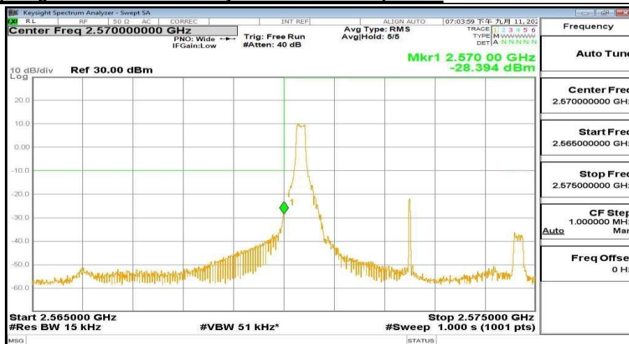
2565MHz-2575MHz_FreqLow_BW(_5MHz)_RB(1@0)_QPSK_Band38
