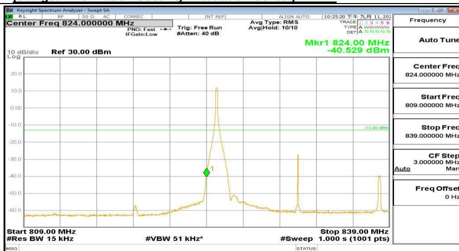
809MHz-839MHz_FreqLow_BW(15MHz)_RB(1@0)_QPSK_Band26
