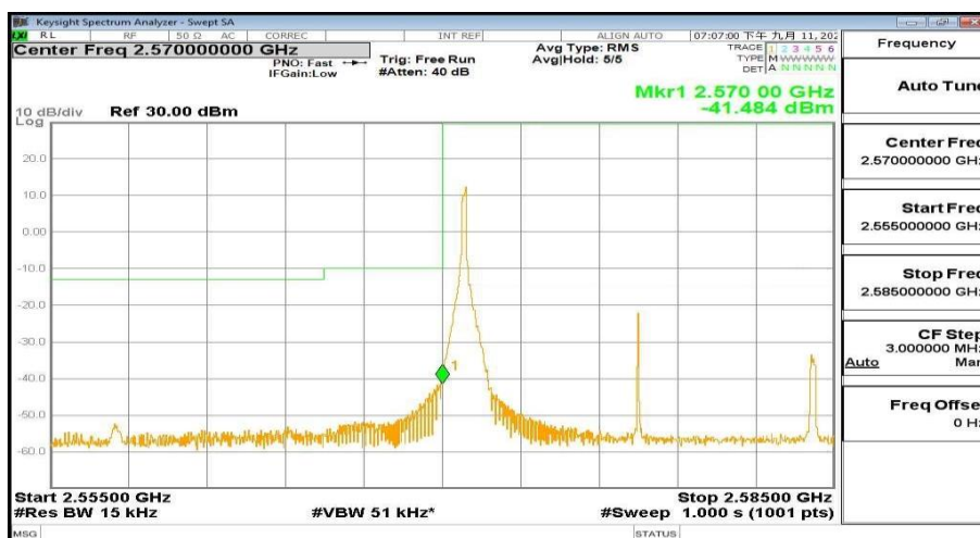
2555MHz-2585MHz_FreqLow_BW(_15MHz)_RB(1@0)_QPSK_Band38
