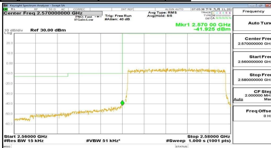
2560MHz-2580MHz_FreqLow_BW(_10MHz)_RB(50@0)_QPSK_Band38
