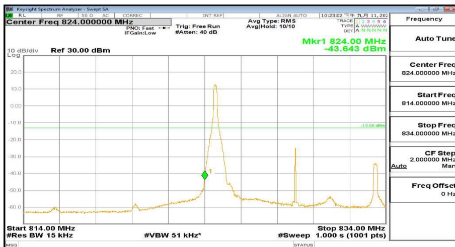
814MHz-834MHz_FreqLow_BW(_10MHz)_RB(1@0)_QPSK_Band26
