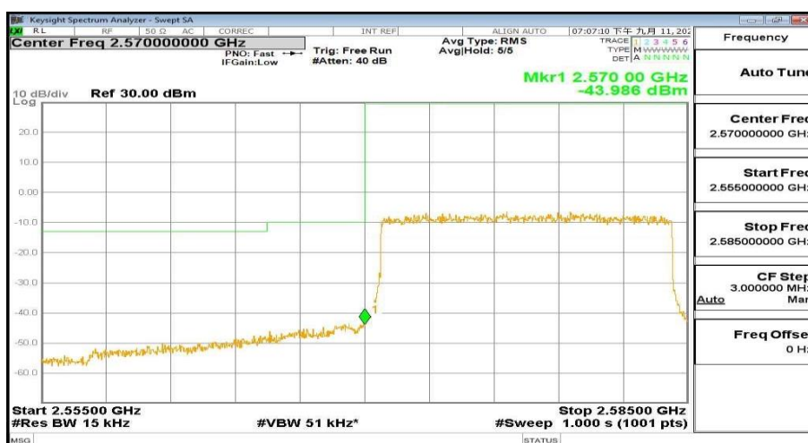
2555MHz-2585MHz_FreqLow_BW(_15MHz)_RB(75@0)_QPSK_Band38
