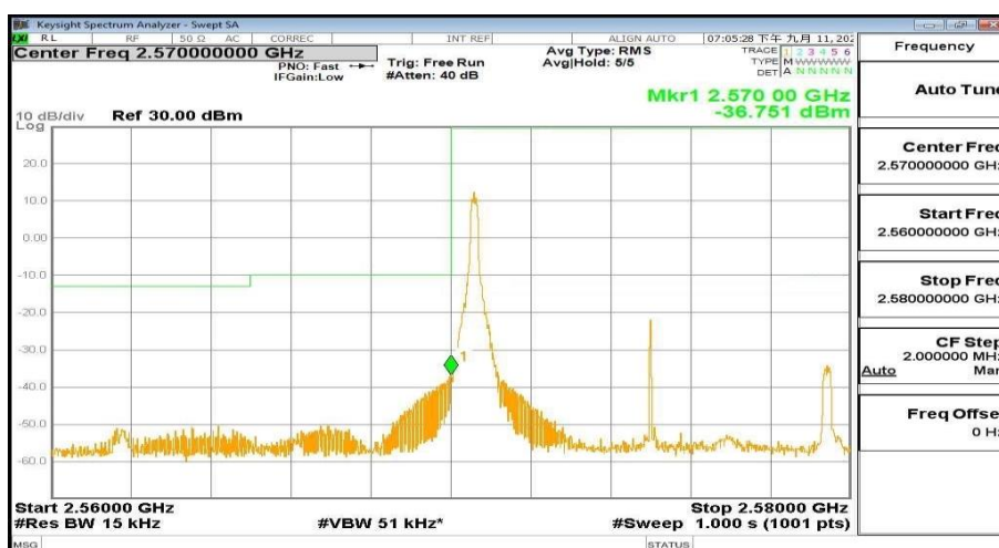
2560MHz-2580MHz_FreqLow_BW(_10MHz)_RB(1@0)_QPSK_Band38
