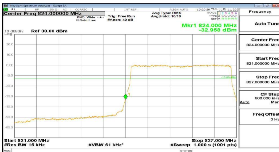
821MHz-827MHz_FreqLow_BW(_3MHz)_RB(15@0)_QPSK_Band26
