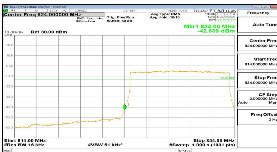
814MHz-834MHz_FreqLow_BW(_10MHz)_RB(50@0)_QPSK_Band26
