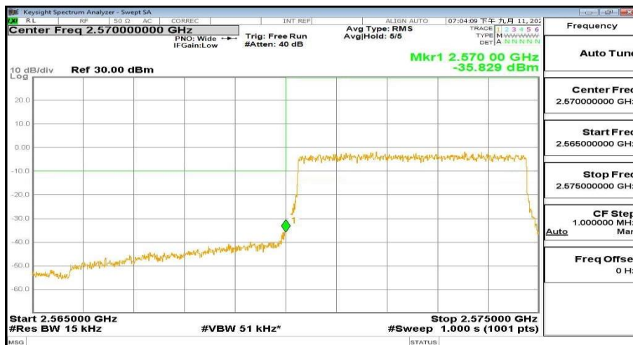
2565MHz-2575MHz_FreqLow_BW(_5MHz)_RB(25@0)_QPSK_Band38
