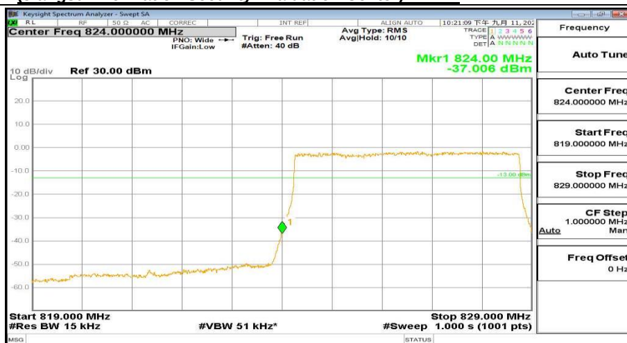
819MHz-829MHz_FreqLow_BW(_5MHz)_RB(25@0)_QPSK_Band26
