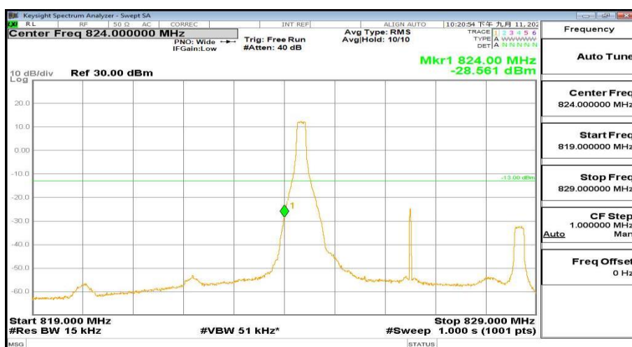
819MHz-829MHz_FreqLow_BW(_5MHz)_RB(1@0)_QPSK_Band26
