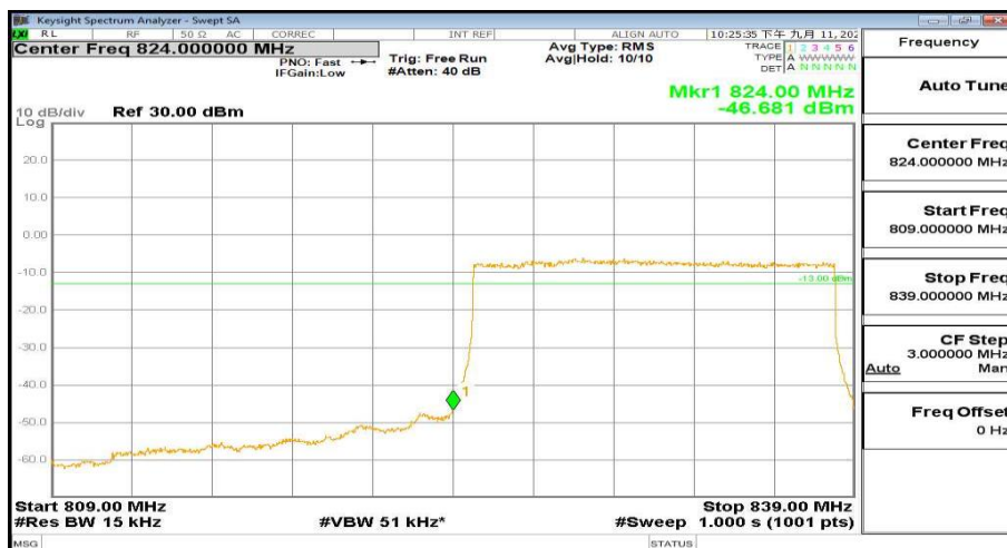
809MHz-839MHz_FreqLow_BW(15MHz)_RB(75@0)_QPSK_Band26
