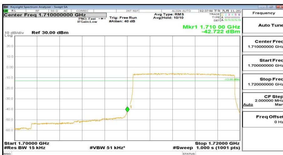
1700MHz-1720MHz_FreqLow_BW(10MHz)_RB(50@0)_QPSK_Band4
