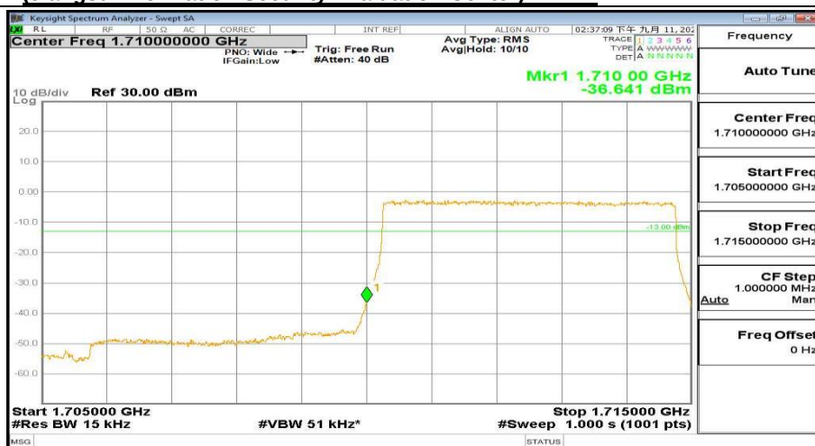
1705MHz-1715MHz_FreqLow_BW(5MHz)_RB(25@0)_QPSK_Band4
