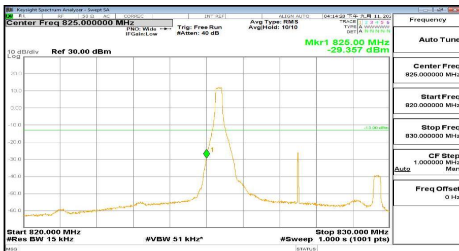
820MHz-830MHz_FreqLow_BW(_5MHz)_RB(1@0)_QPSK_Band5
