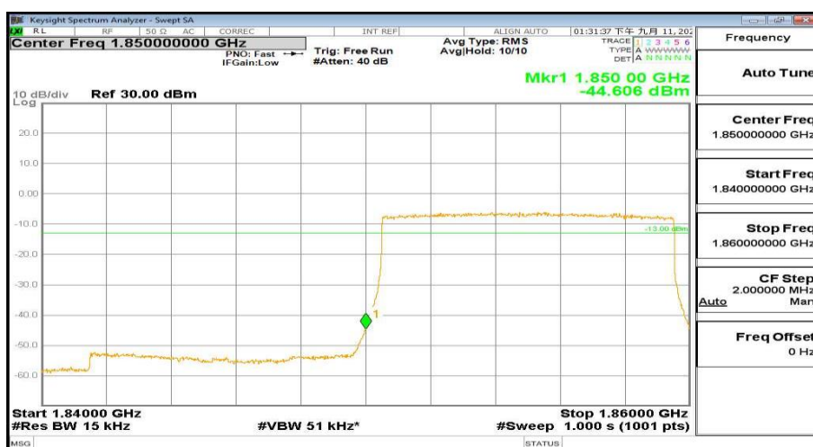
1840MHz-1860MHz_FreqLow_BW(10MHz)_RB(50@0)_QPSK_Band2
