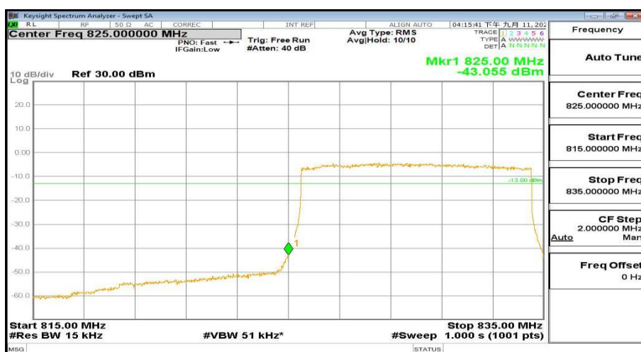
815MHz-835MHz_FreqLow_BW(_10MHz)_RB(50@0)_QPSK_Band5
