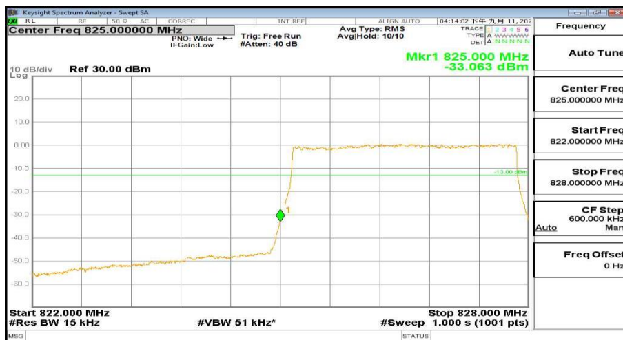
822MHz-828MHz_FreqLow_BW(_3MHz)_RB(15@0)_QPSK_Band5
