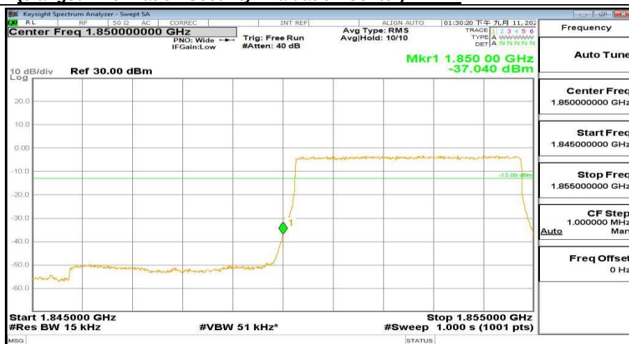
1845MHz-1855MHz_FreqLow_BW(5MHz)_RB(25@0)_QPSK_Band2
