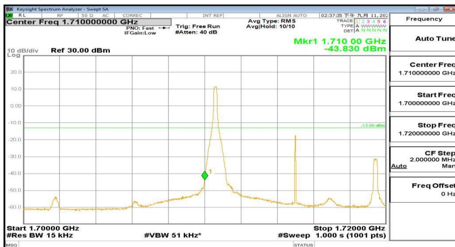
1700MHz-1720MHz_FreqLow_BW(10MHz)_RB(1@0)_QPSK_Band4
