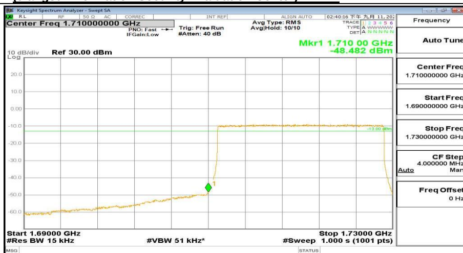
1690MHz-1730MHz_FreqLow_BW(_20MHz)_RB(100@0)_QPSK_Band4
