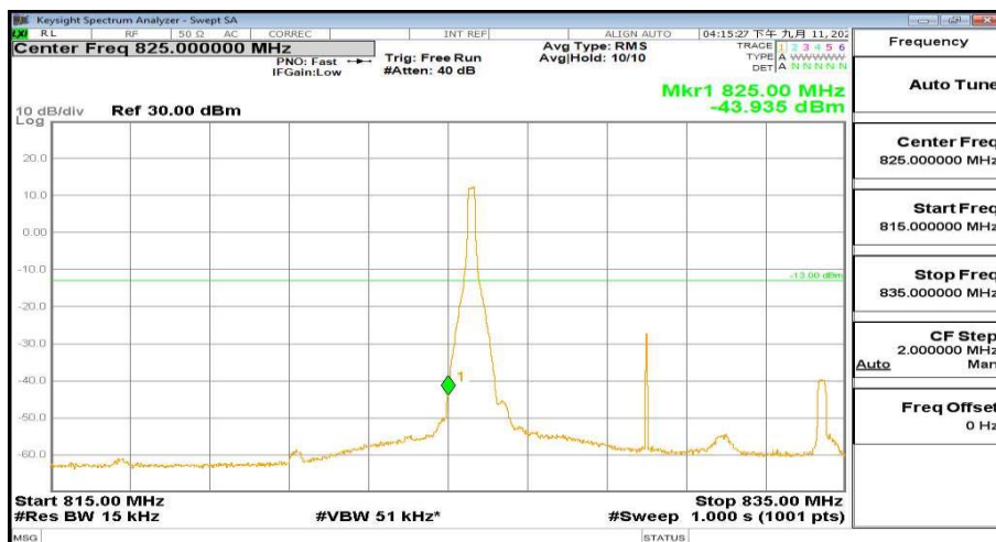
815MHz-835MHz_FreqLow_BW(_10MHz)_RB(1@0)_QPSK_Band5
