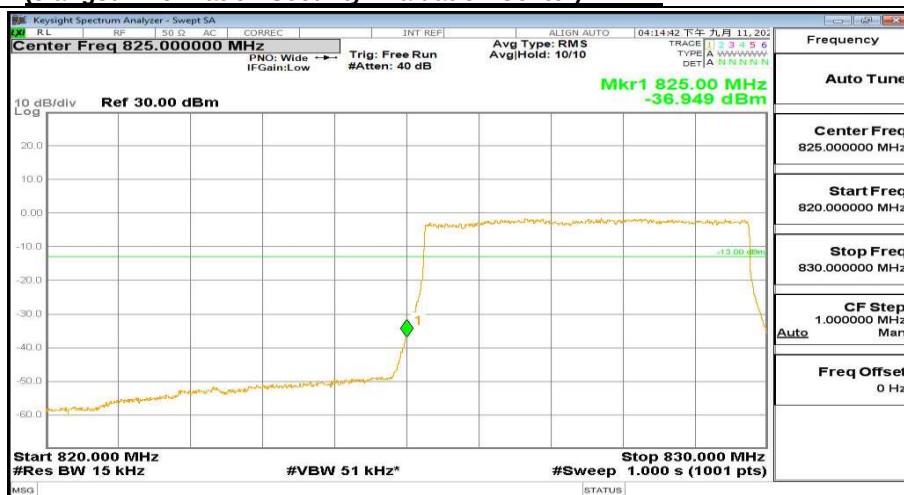
820MHz-830MHz_FreqLow_BW(_5MHz)_RB(25@0)_QPSK_Band5
