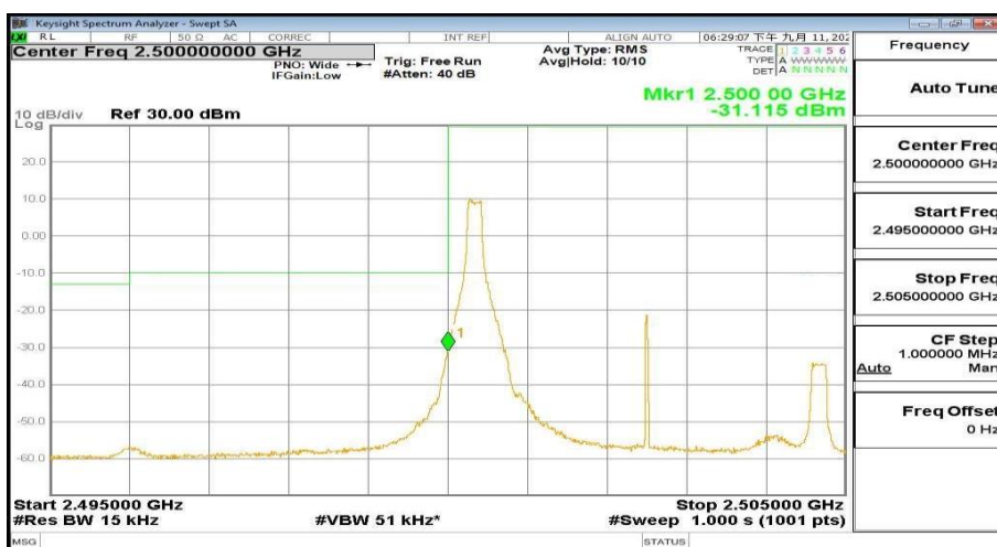
2495MHz-2505MHz_FreqLow_BW( 5MHz)_RB(1@0)_QPSK_Band7
