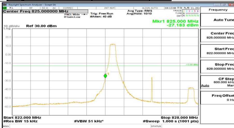
822MHz-828MHz_FreqLow_BW(_3MHz)_RB(1@0)_QPSK_Band5
