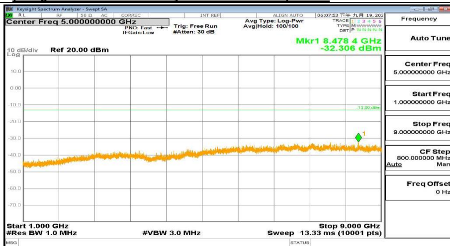
WCDMA Band5 Channel-4233 1GHz-9GHz
