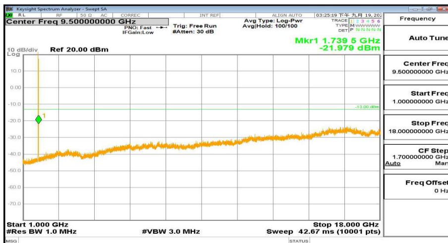
WCDMA Band4 Channel-1413 1GHz-18GHz
