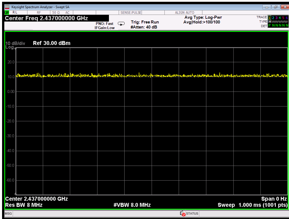
802.11n40 mode(Ant 1)
