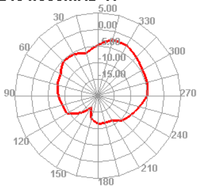
2484.000MHz H
