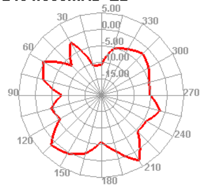
2484.000MHz E2
