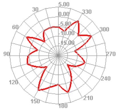
2441.000MHz E1
