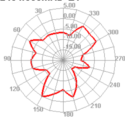
2484.000MHz E1
