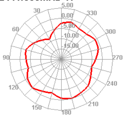
2441.000MHz H
