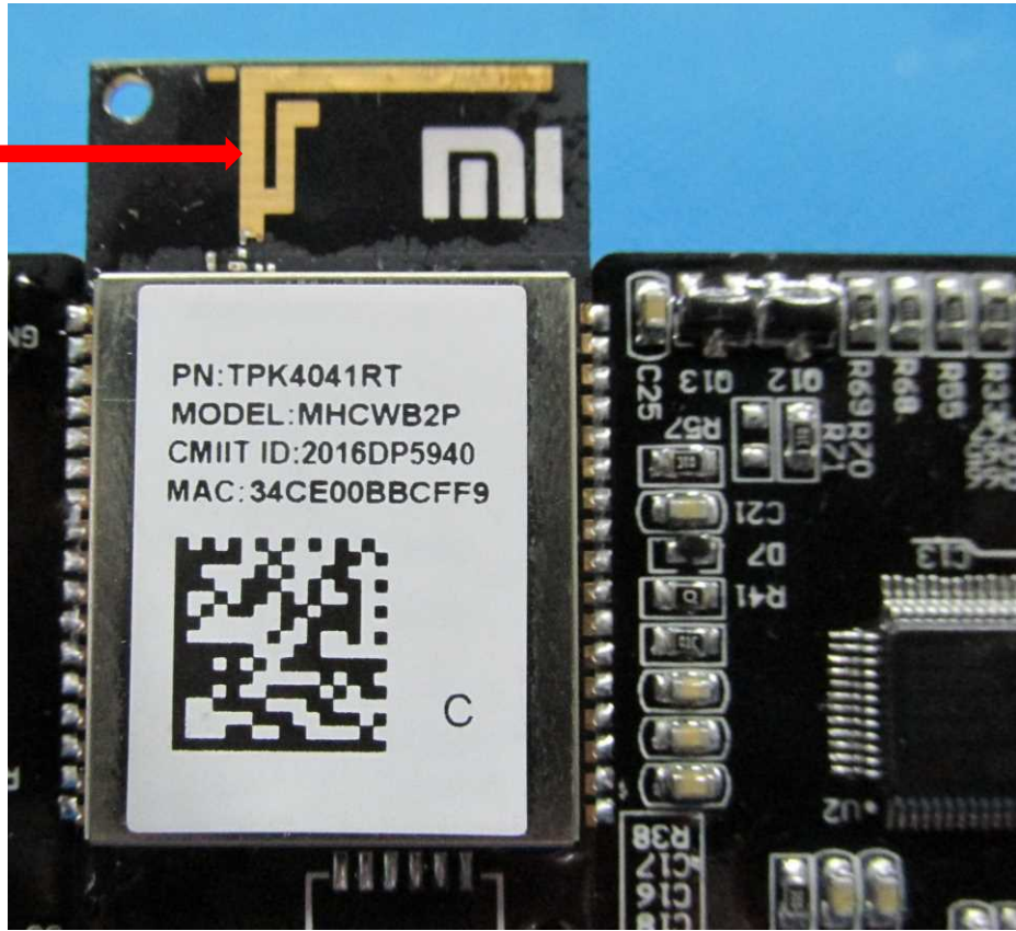
2.4GHz Wi-Fi RF Module
