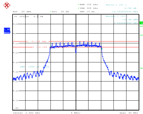
g_2462MHz_Chain 0 16.160MHz
