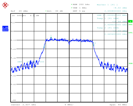
g_2437MHz_Chain 0 17.000MHz
