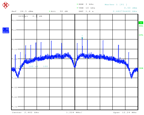
b_2462MHz_Chain 0 0.50dBm/3kHz
