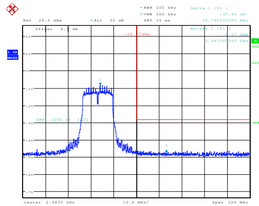
g_2462MHz_Chain 0 37.84dB
