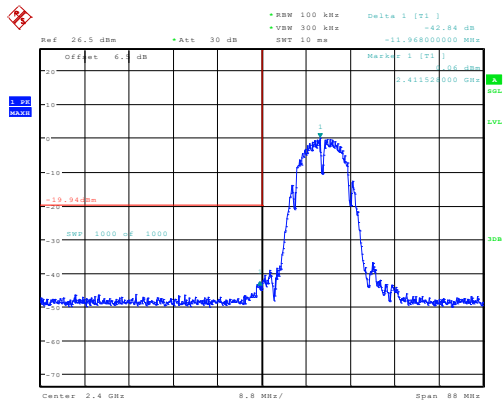
b_2412MHz_Chain 0 42.84dB
