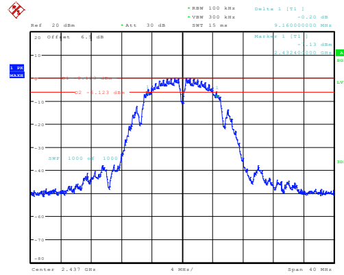
b_2437MHz_Chain 0 9.160MHz
