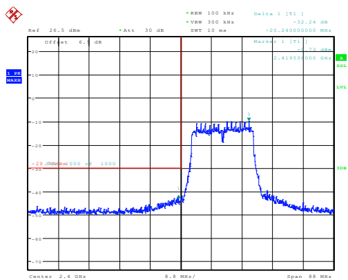
n20_2412MHz_Chain 0 32.24dB
