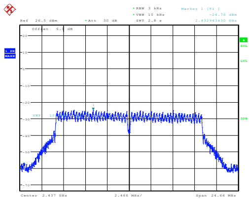
g_2437MHz_Chain 0 -24.76dBm/3kHz
