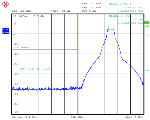
GFSK_Low 57.31dB
