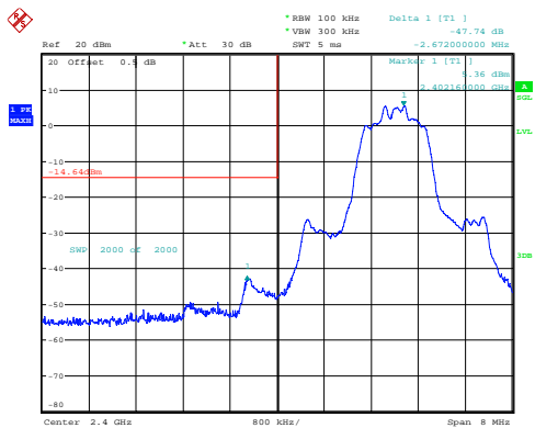
\pi/4 -DQPSK_Low 47.74dB
