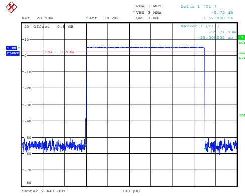
GFSK_Hopping_DH3 1.671ms
