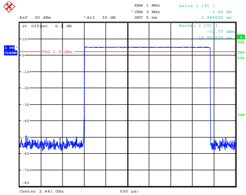
GFSK_Hopping_DH5 2.945ms
