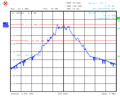
GFSK_Middle 0.897MHz
