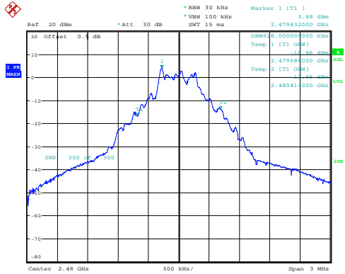
GFSK_High 0.828MHz
