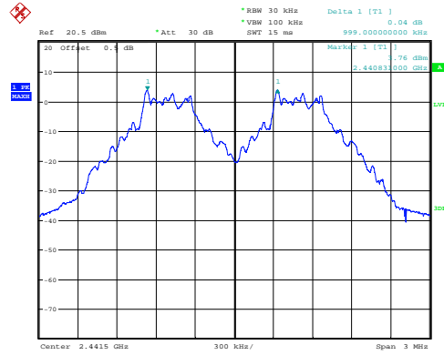
GFSK_Middle 0.999MHz
