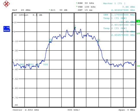
\pi/4 -DQPSK_Low 1.170MHz
