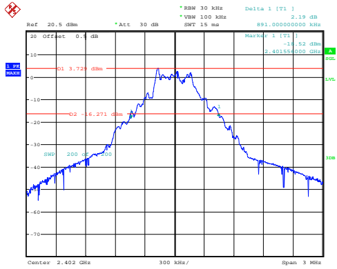
GFSK_Low 0.891MHz
