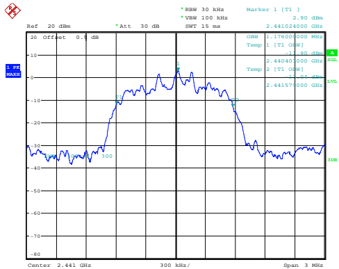
\pi/4 -DQPSK_Middle 1.176MHz
