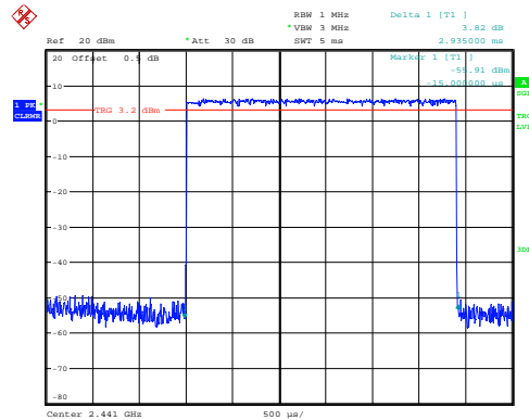
\pi/4 -DQPSK_Hopping_2DH5 2.935ms
