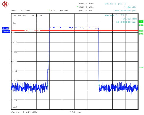
GFSK_Hopping_DH1 0.409ms
