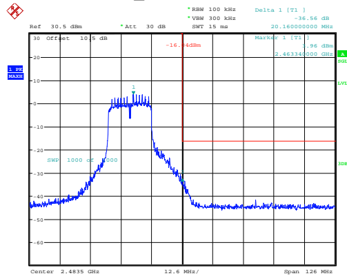
n20_2462MHz 36.56dB
