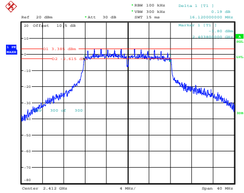
g_2412MHz 16.120MHz
