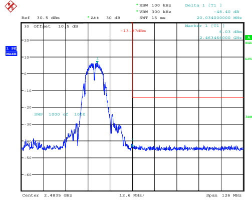
b_2462MHz 48.40dB
