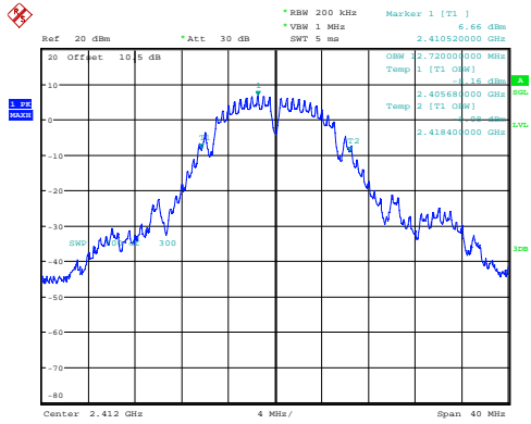
b_2412MHz 12.720MHz
