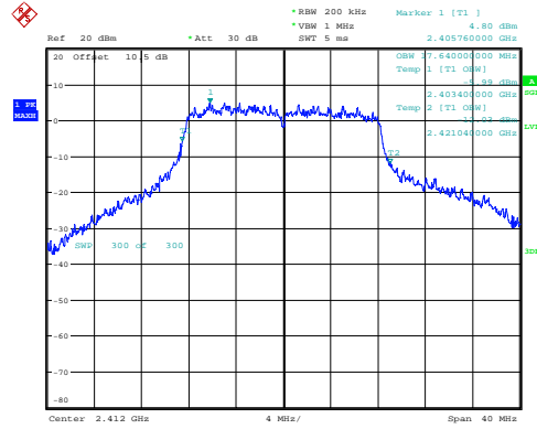
g_2412MHz 17.640MHz
