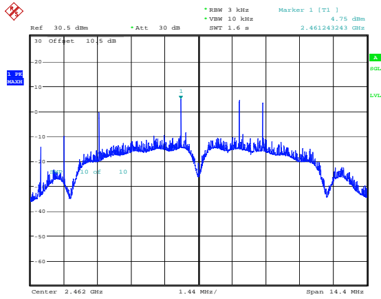
b_2462MHz 4.75dBm/3kHz
