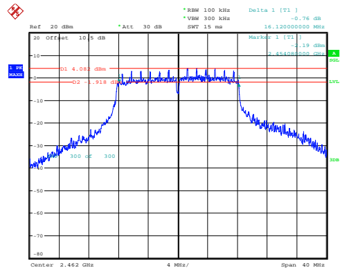
g_2462MHz 16.120MHz
