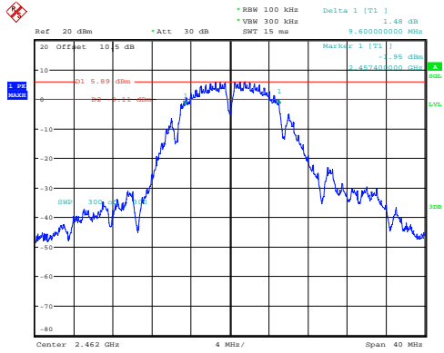
b_2462MHz 9.600MHz
