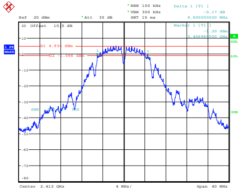
b_2412MHz 9.600MHz
