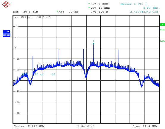
b_2412MHz 3.07dBm/3kHz
