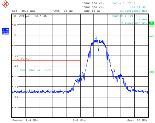
b_2412MHz 36.91dB
