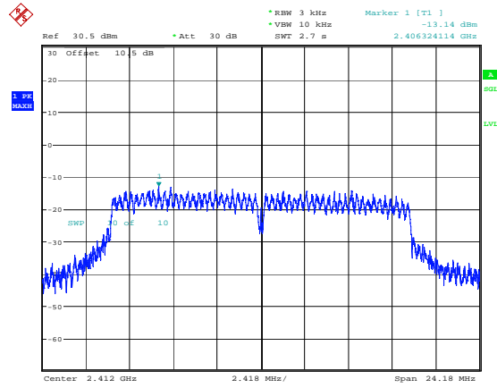
g_2412MHz -13.14dBm/3kHz
