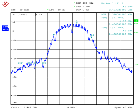
b_2462MHz 12.320MHz
