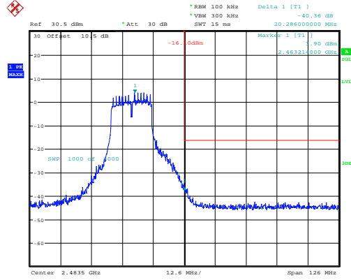
g_2462MHz 40.36dB
