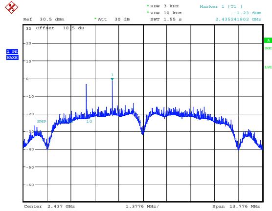
b_2437MHz -1.23dBm/3kHz
