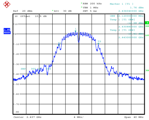
b_2437MHz 12.120MHz
