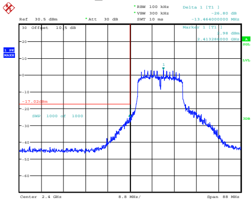
n20_2412MHz 26.80dB
