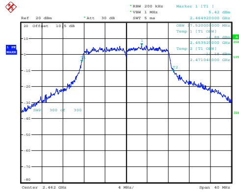
g_2462MHz 17.520MHz
