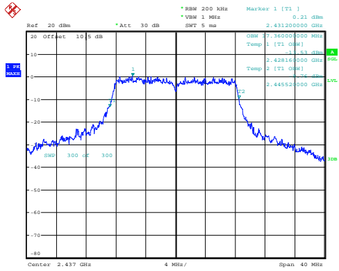
g_2437MHz 17.360MHz
