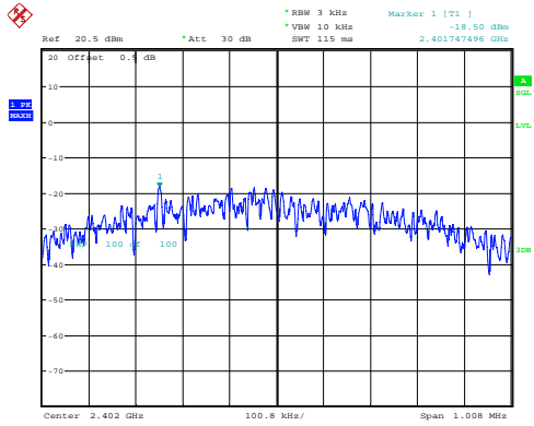
Low -18.50dBm/3kHz
