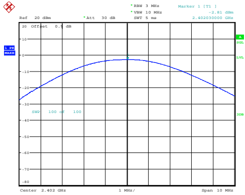
Low -2.81dBm
