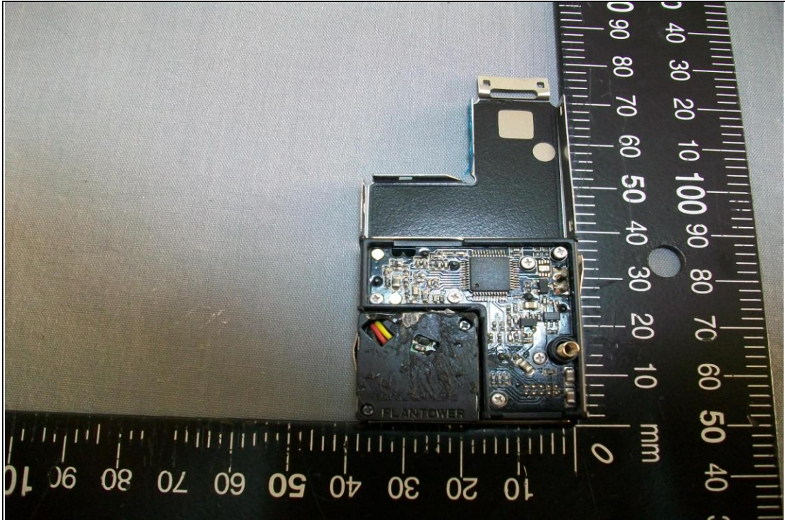
< PCB6-F >
