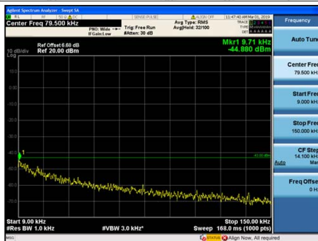
GPRS1900_661
