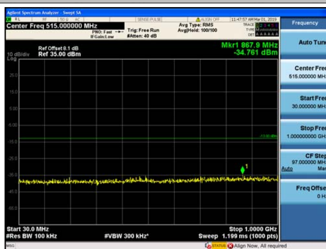
GPRS1900_661
