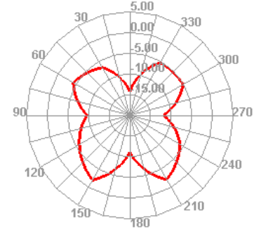
2400.000MHz E2
