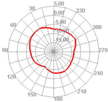
2450.000MHz H
