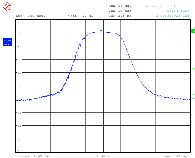
RMS detector is for AV value
