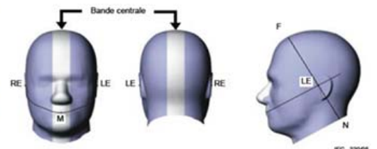
Illustration du fantôme donnant les points de référence des oreilles, RE et LE, le point de référence de la bouche, M, la ligne de référence H-F et la bande centrale
