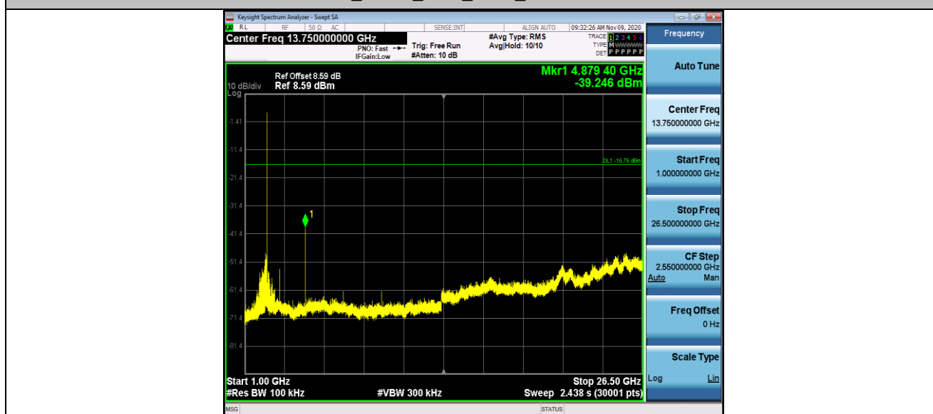
BLE_BT5.0_Ant1_2480_0~Reference
