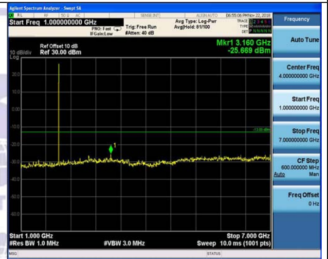
1GHz~7GHz
