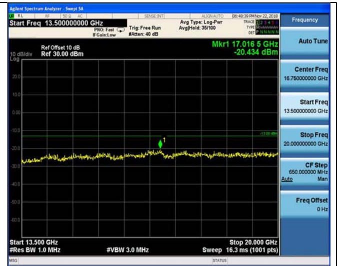
13.5GHz~20GHz 810
