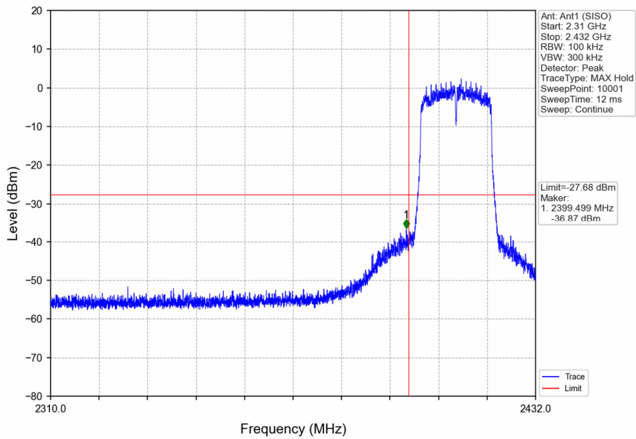
802.11n(HT20)_LCH_2412MHz_Ant1 (SISO)_NTNV
