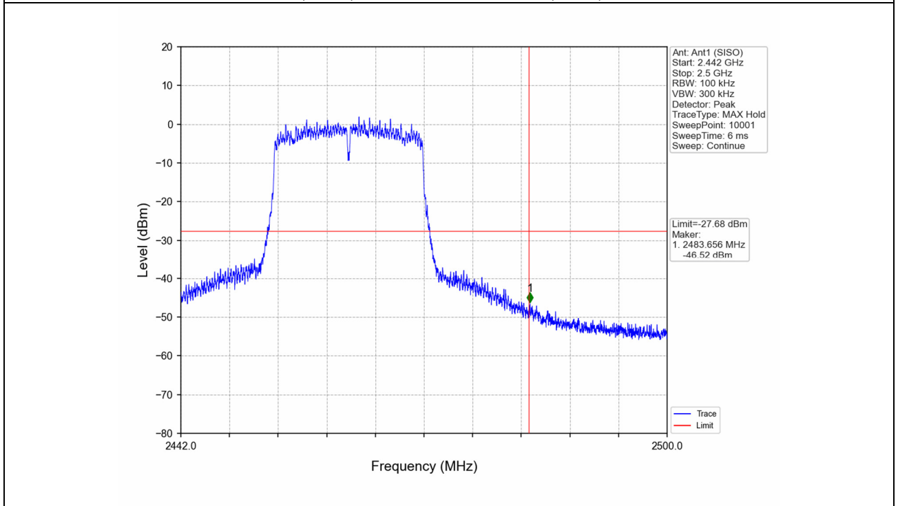
802.11n(HT20)_HCH_2462MHz_Ant1 (SISO)_NTNV
