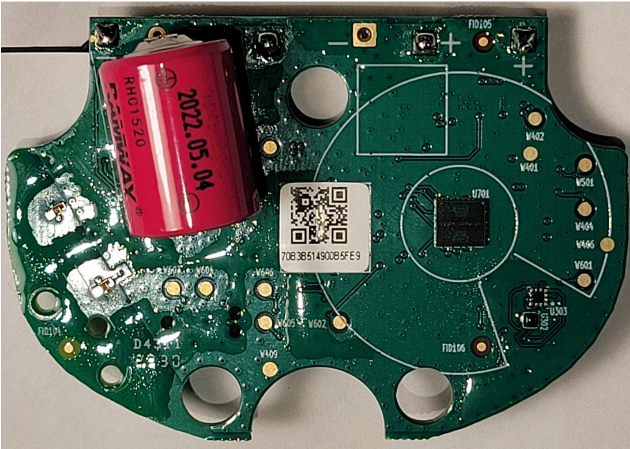
PCB top
