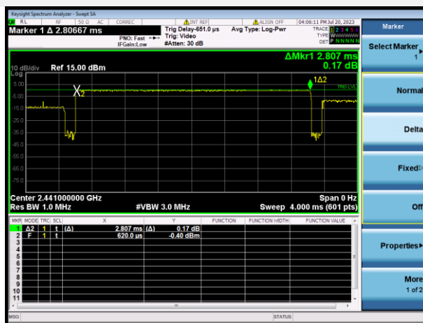
GFSK DH5
