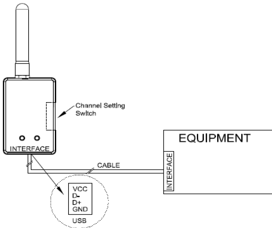
KTX433-USB Interface & Cable
