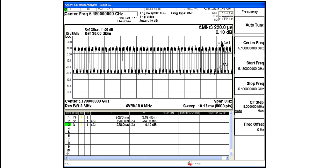
11AX20MIMO_Ant2_5180
