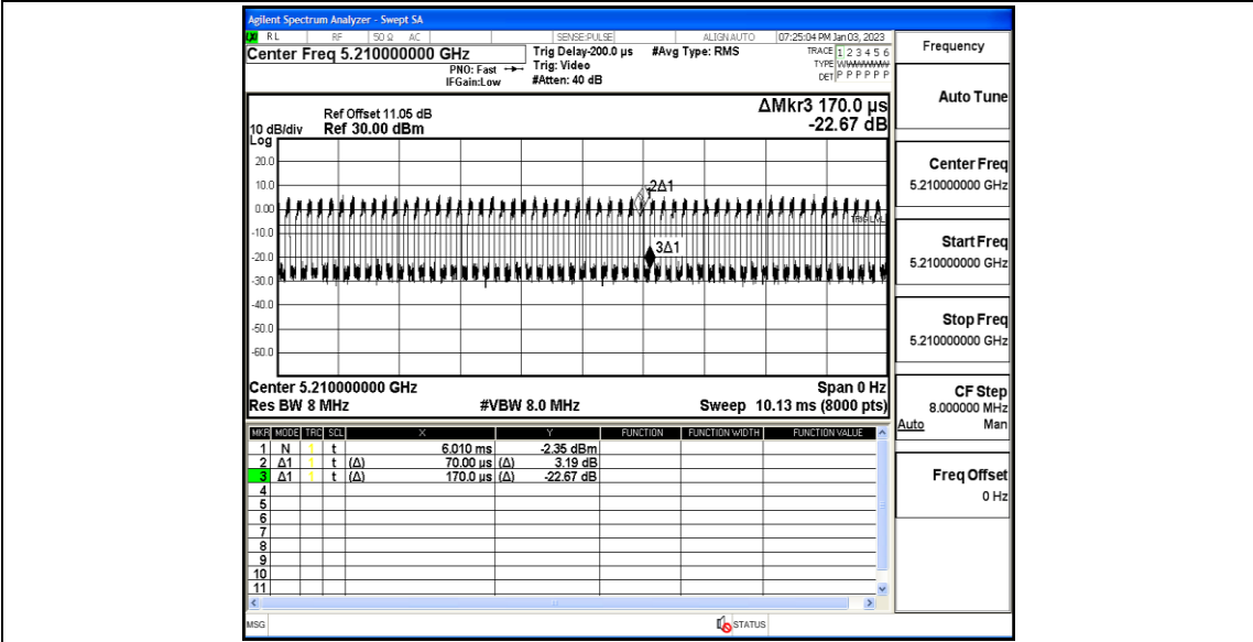
11AX80MIMO_Ant2_5210
