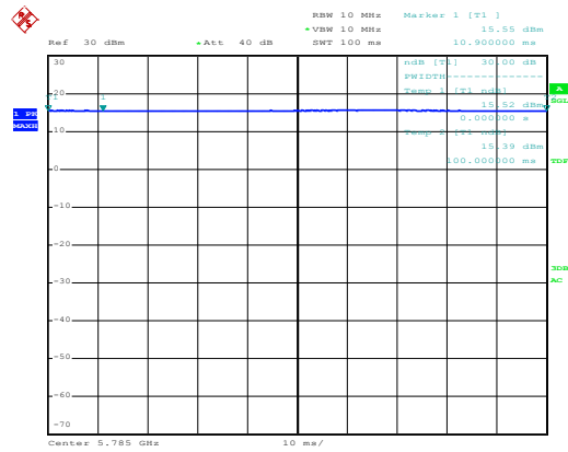
IEEE 802.11a
