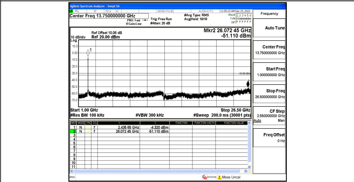
11N40MIMO_Ant2_2437_0~Reference
